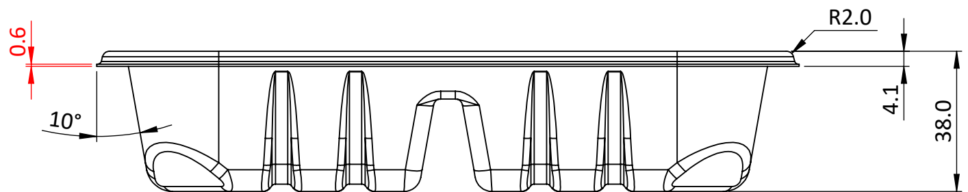
ELEVATION
