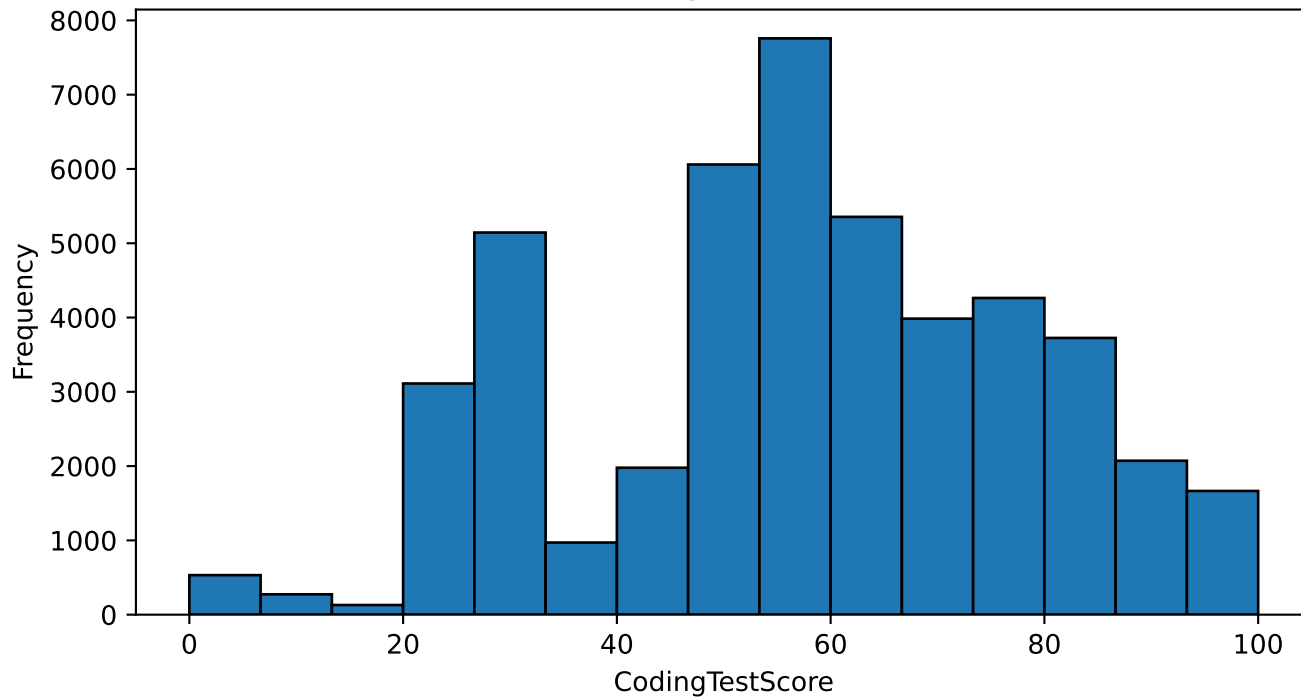
CodingTestScore
