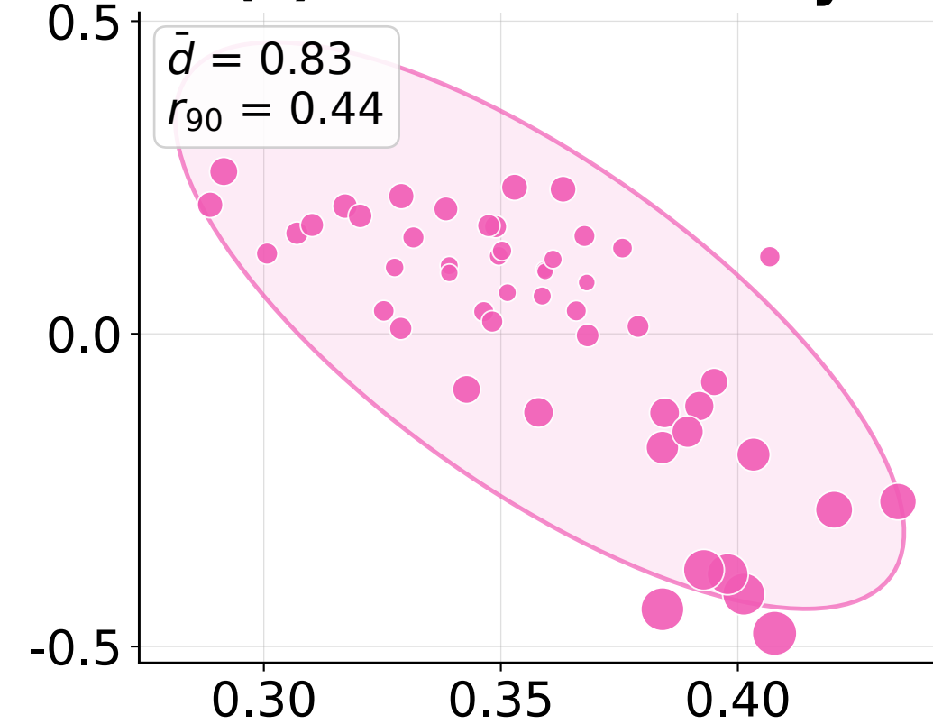
(f) Web
