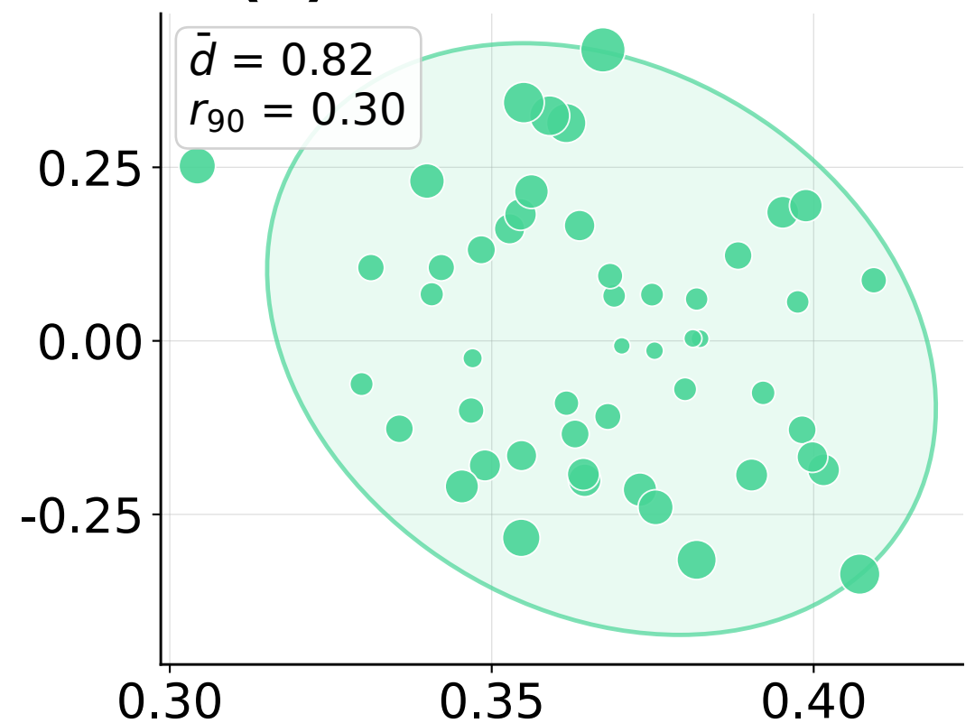
(d) Chatbot-Finance
