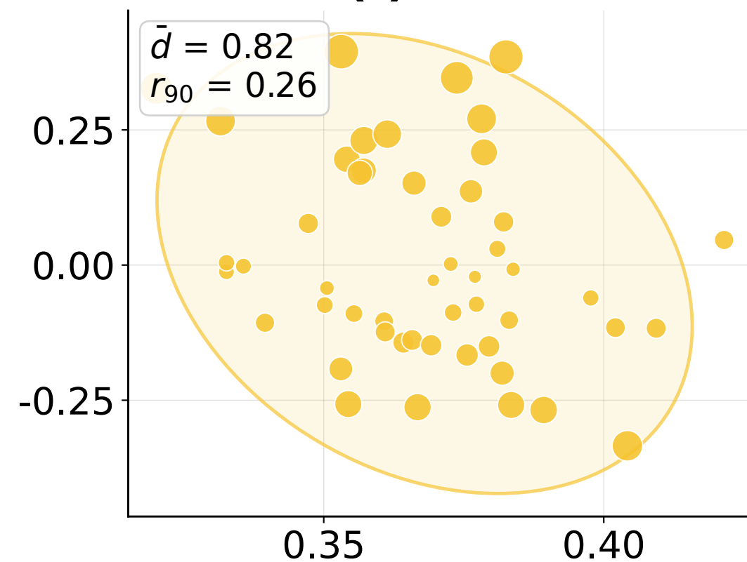
(f) Web
