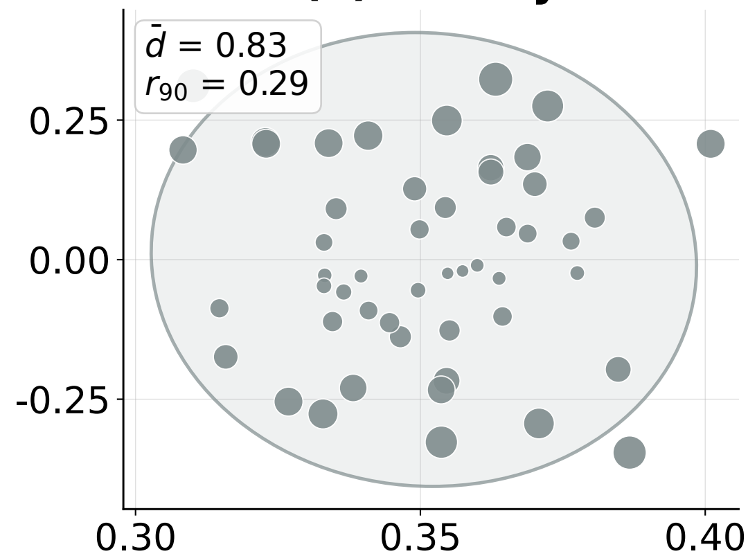
(d) Chatbot-Finance
