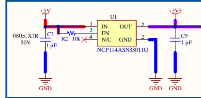
3V3 LDO
