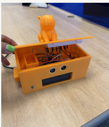
THE WIRING
