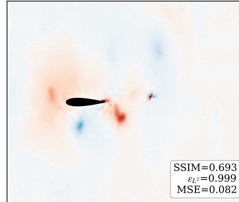
JEPA KRR
