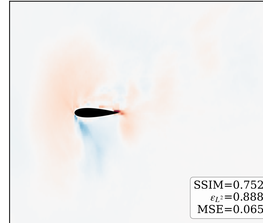
POD KRR
