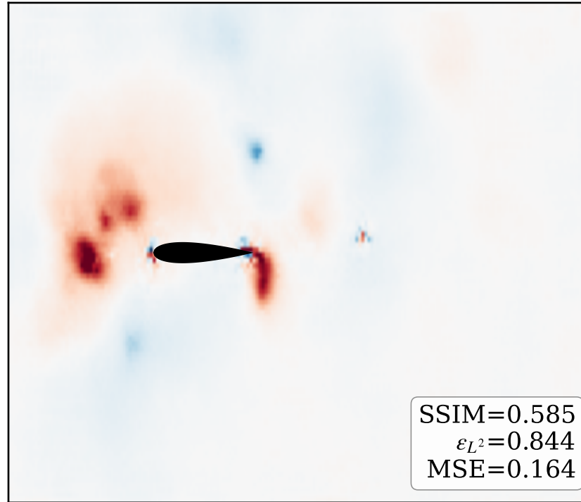
JEPA
