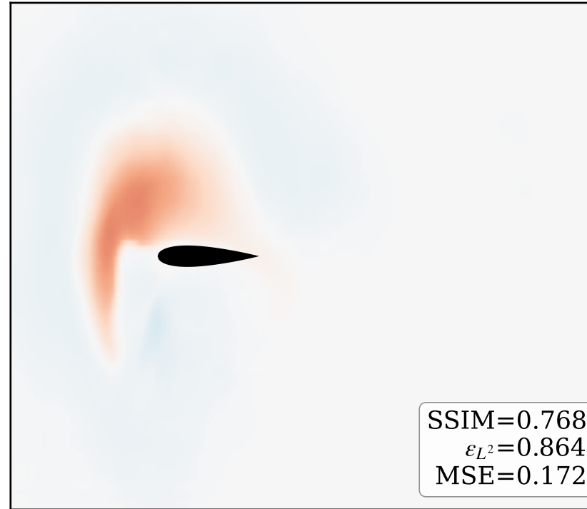
Fukami AE
