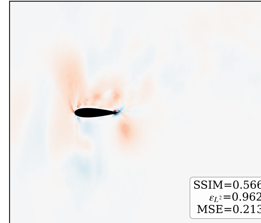
POD KRR
