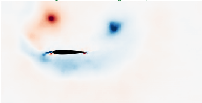
predictive (JEPA)
