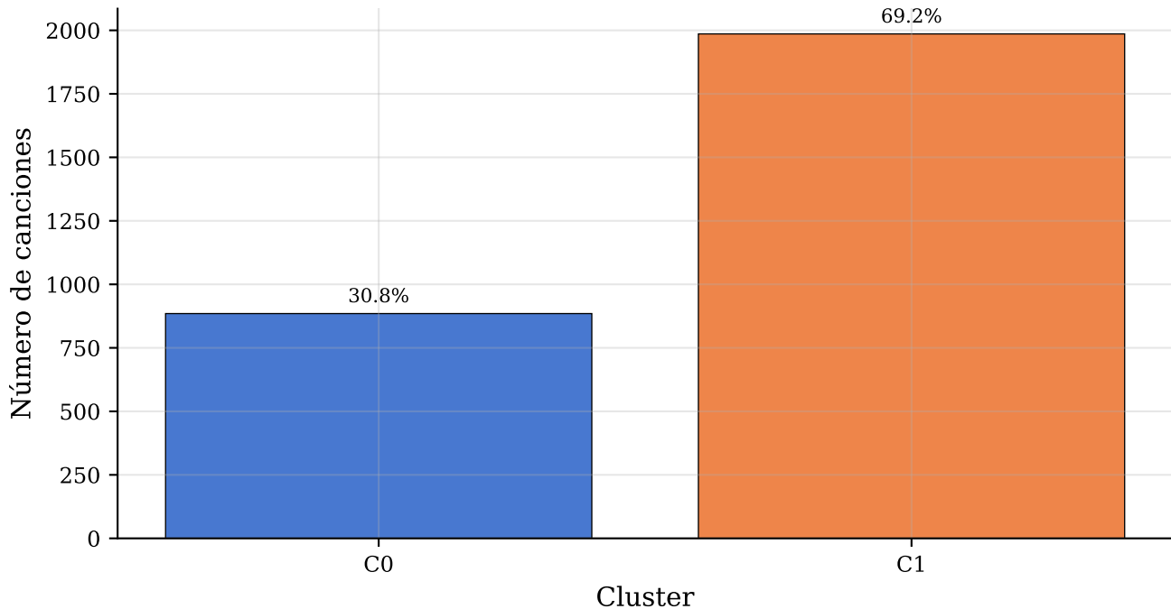
Distribución de clusters --- HDBSCAN K = 2 , Musical (13D)
