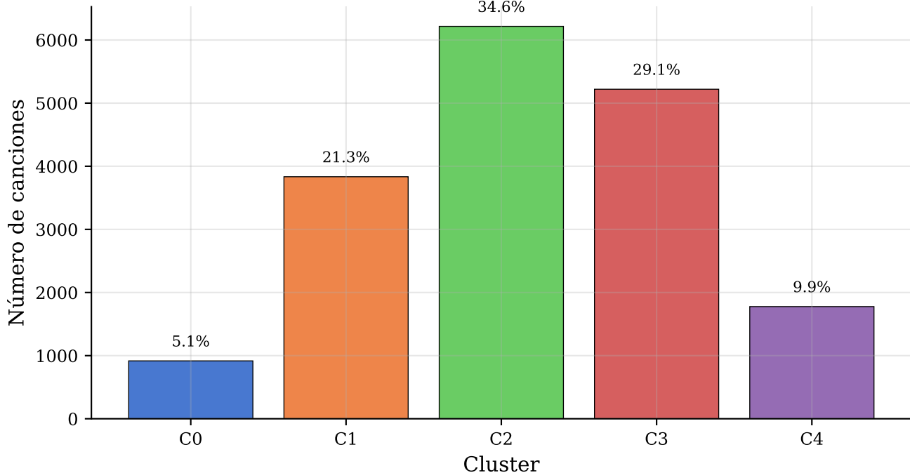
Distribución de clusters --- Kmeans K = 5 , Semántico (384D)
