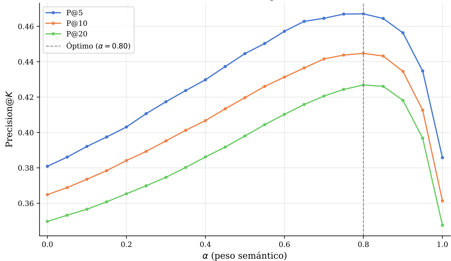
Precisión en función del peso de fusión
