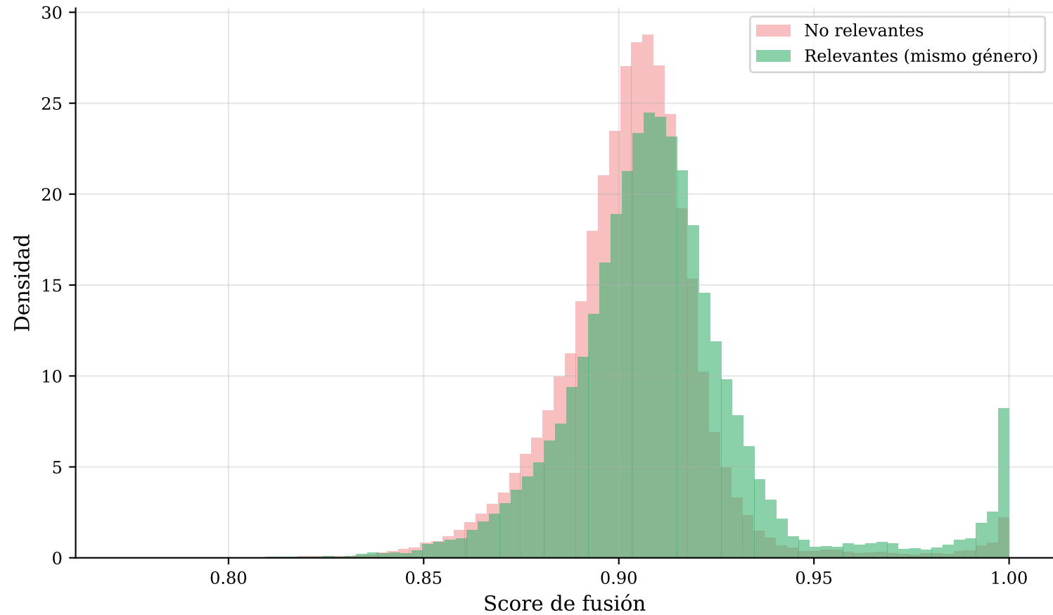
Distribución de scores: relevantes vs. no relevantes
