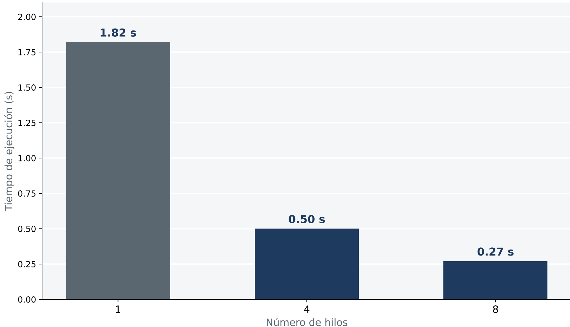
Tiempo de ejecución vs número de hilos
