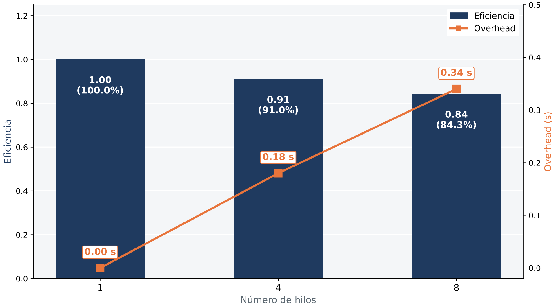
Eficiencia y Overhead vs número de hilos
