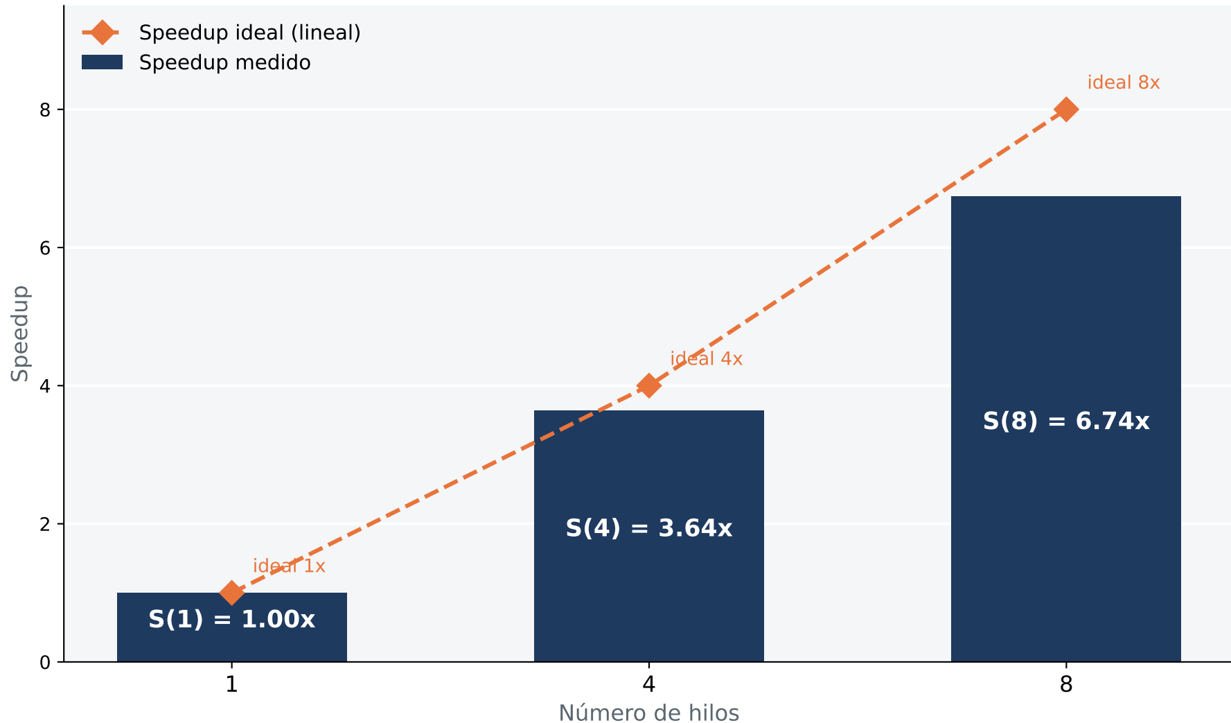
Speedup vs número de hilos
