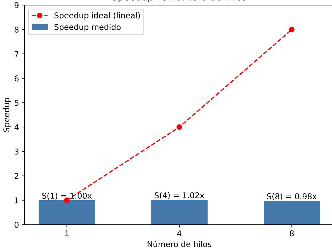
Speedup vs número de hilos
