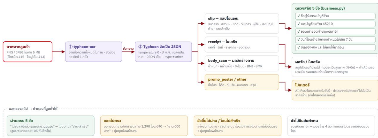
รูปที่ 4 — การอ่านภาพและตรวจสอบสลิปด้วยโค้ด
