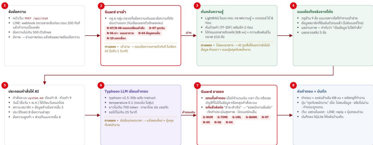
รูปที่ 2 — การทำงานของแชทบอท — 1 ข้อความผ่าน 8 ขั้นตอน
