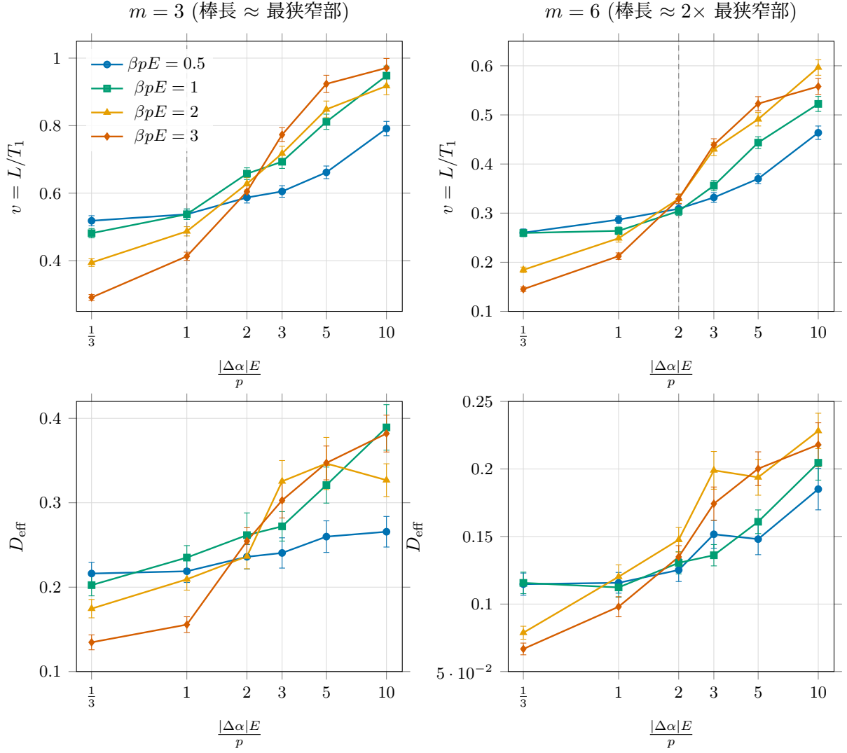
図1 平均速度 v = L/T_1 (上段) と有効拡散係数 D_{\text{eff}} (下段) の \delta = |\Delta\alpha|E/p 依存性. 左列が m = 3 , 右列が m = 6 . 記号は永久双極子と熱エネルギーの比 \beta p E を表す. 誤差棒は初通過時間のブートストラップ標準誤差, 破線は傾いた向きが最狭部に収まる幾何閾値 ( m = 3 で \delta = 1 , m = 6 で \delta = 2 ) を示す.
