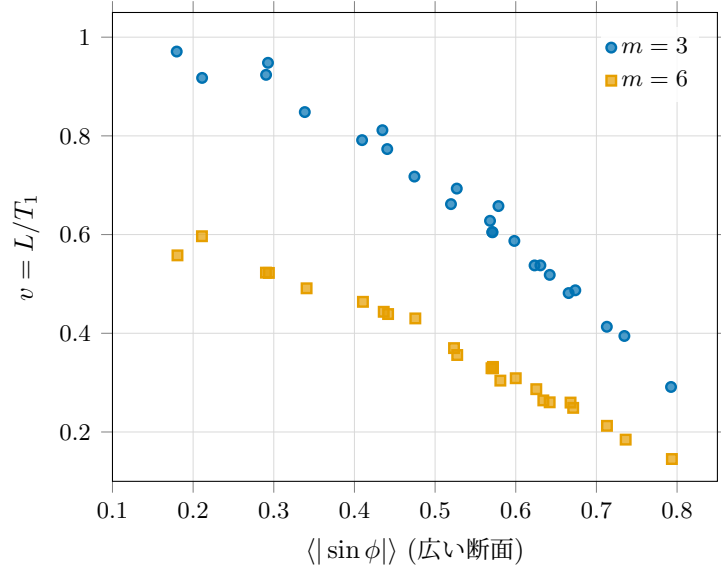
図5 広い断面での \langle |\sin \phi| \rangle ( y 軸方向への射影の指標) と平均速度 v = L/T_1 の関係 (全 48 条件). 棒長ごとに単調減少の帯に乗り, 棒の向きが輸送を律速することを示す.
