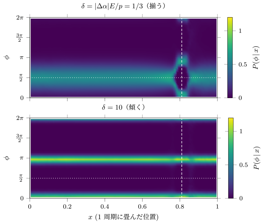
Fig. 6 (x, \phi) 占有マップ P(\phi | x)
