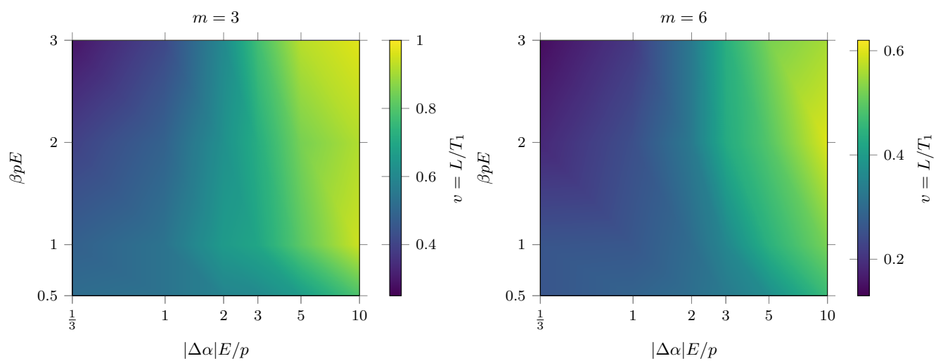
Fig. 5 分離の動作マップ v(|\Delta\alpha|E/p, \beta pE)
