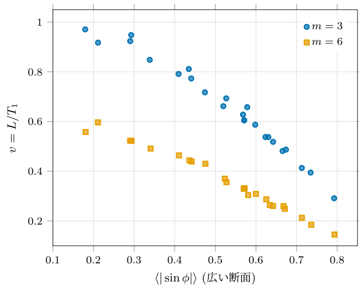
Fig. 4 配向 \rightarrow 輸送の対応
