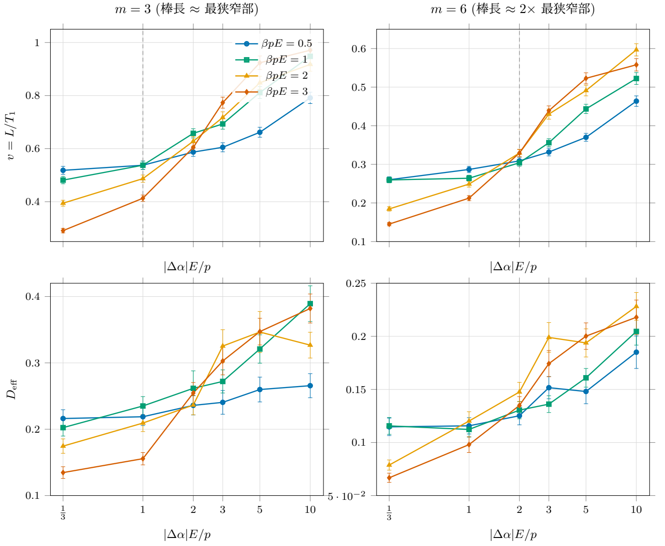
Fig. 1 主結果: v と D_{\text{eff}} の |\Delta\alpha|E/p 依存性
