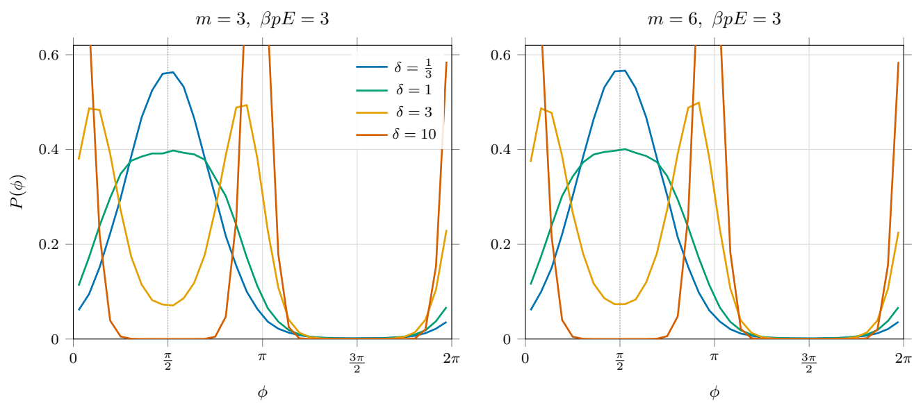
Fig. 3 機構: 配向分布 P(\phi)
