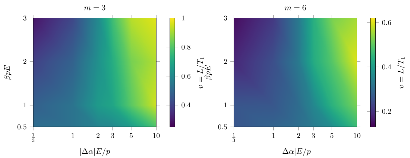
図6 パラメータ平面 (\delta, \beta p E) 上の平均速度 v = L/T_1 (左 m = 3 , 右 m = 6 ). 同じ動作点でも棒長によって v が分かれることが, 移動度の差による分離の動作マップを与える.
