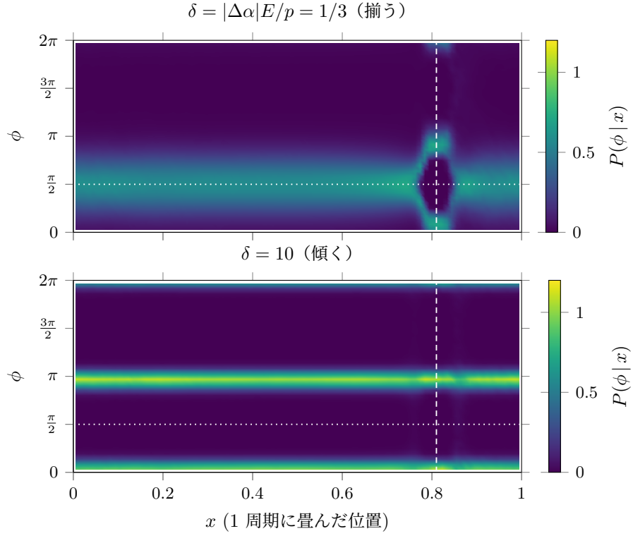
図3 (x, \phi) 占有マップ ( m = 6 , \beta p E = 3 ). 色は各位置 x での条件付き配向分布 P(\phi|x) . 破線は最狭窄部 x \approx 0.81 , 点線は \phi = \pi/2 . \delta = 1/3 (上) では棒は広域で \phi = \pi/2 に揃うが最狭窄部でのみ軸方向に選別され, \delta = 10 (下) では全域で軸方向に傾いて最狭窄部を乱されずに通過する.
