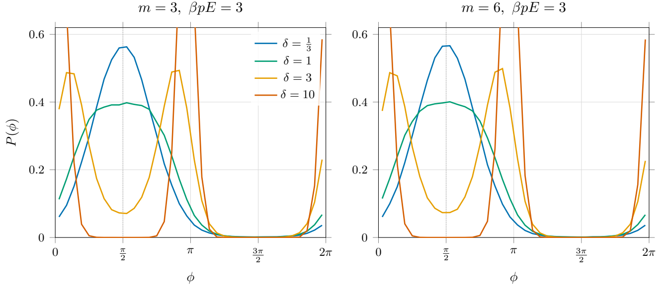
図2 広い断面 ( x \approx 0.20 ) における配向分布 P(\phi) ( m=3 と m=6 , いずれも \beta pE=3 ). \delta が小さいと \phi = \pi/2 (点線) に単峰, 大きいと \phi_1 = \arcsin(1/\delta) 付近 (軸方向) へ移動して二峰化する.
