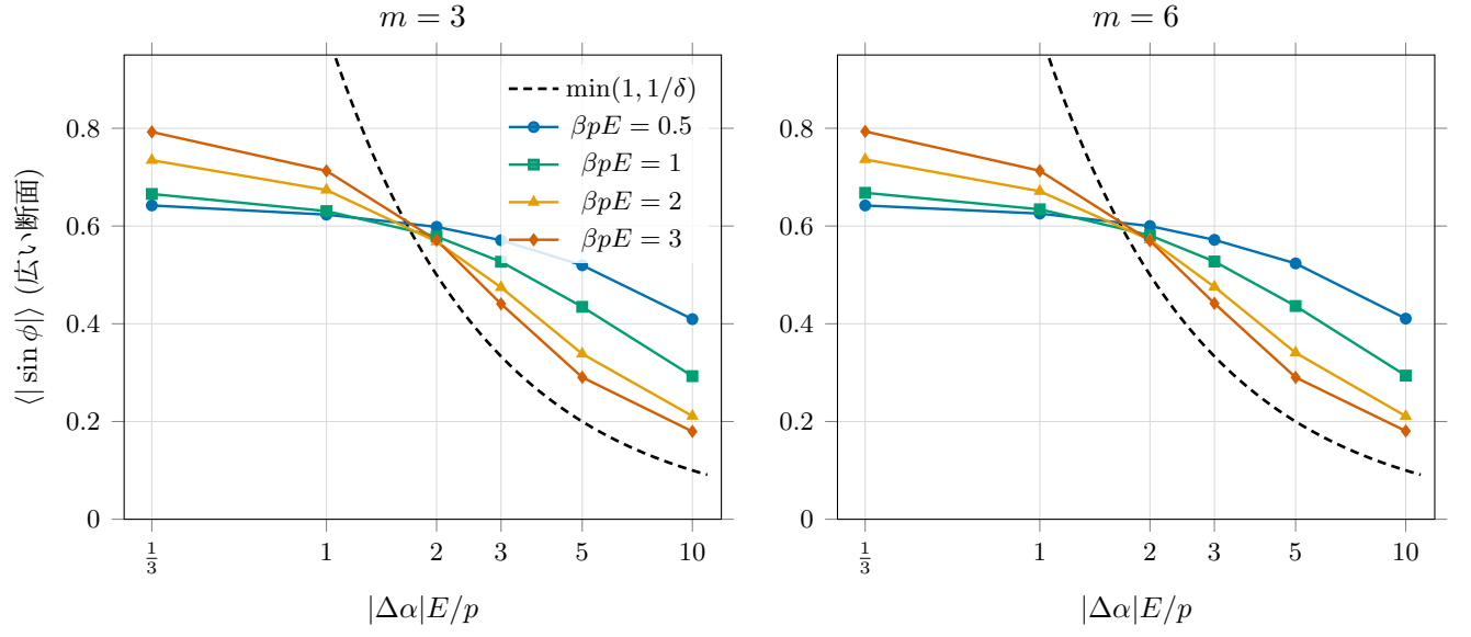
図4 広い断面における占有重み付き \langle |\sin \phi| \rangle の \delta 依存性. 破線は安定配向 \sin \phi_1 = 1/\delta から定まる理論値 \min(1, 1/\delta) .
