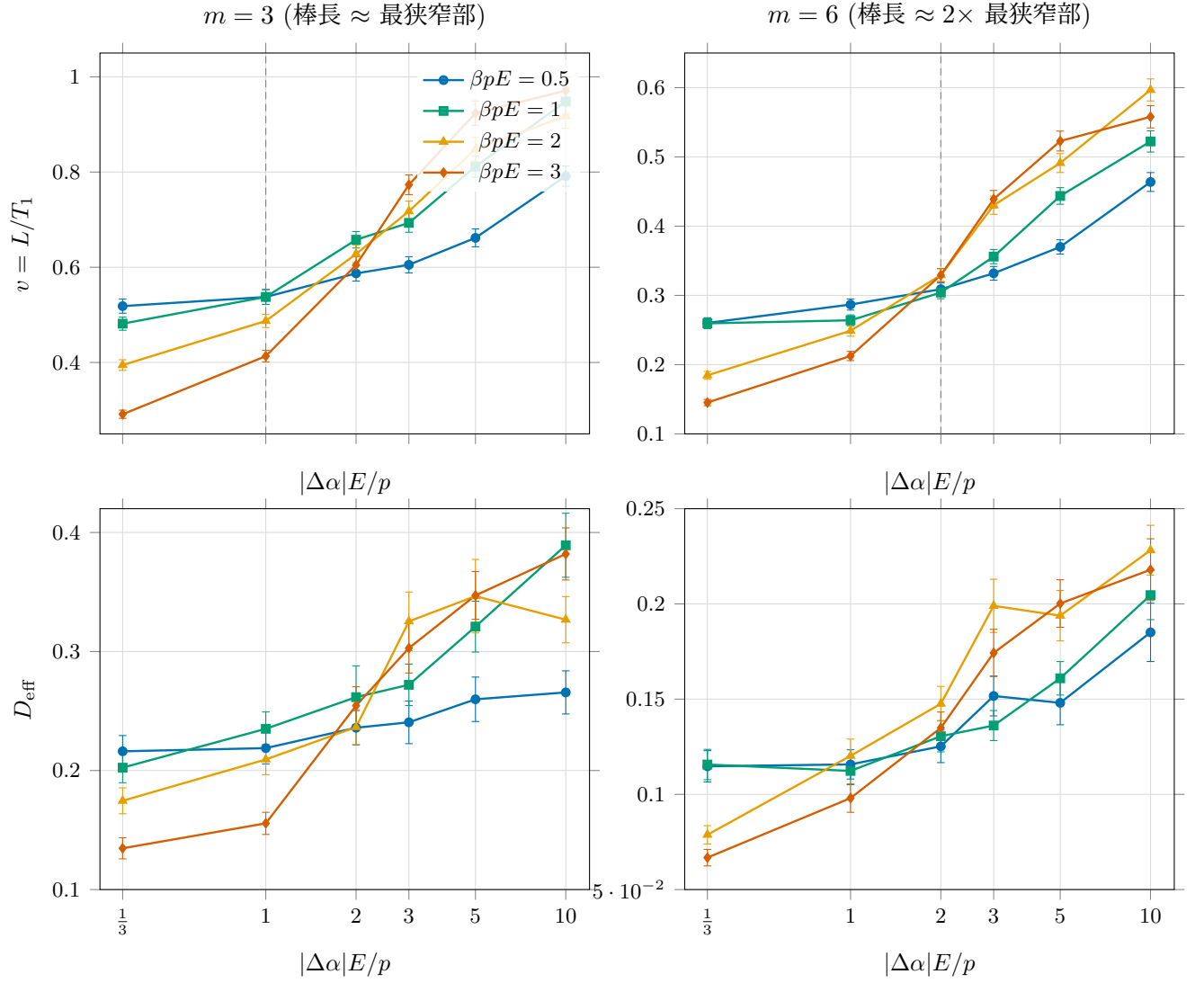
図1 平均速度 v = L/T_1 (上段) と有効拡散係数 D_{\text{eff}} (下段) の \delta = |\Delta\alpha|E/p 依存性. 左列が m = 3 , 右列が m = 6 . 記号は永久双極子と熱エネルギーの比 \beta p E を表す. 誤差棒は初通過時間のブートストラップ標準誤差, 破線は傾いた配向が最狭窄部に収まる幾何閾値 ( m = 3 で \delta = 1 , m = 6 で \delta = 2 ) を示す.
