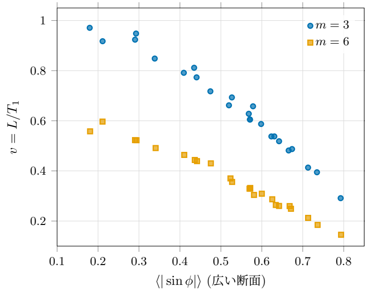
図5 広い断面での \langle |\sin \phi| \rangle (張り出しの指標) と平均速度 v = L/T_1 の関係 (全 48 条件). 棒長ごとに単調減少の帯に乗り, 配向が輸送を律速することを示す.
