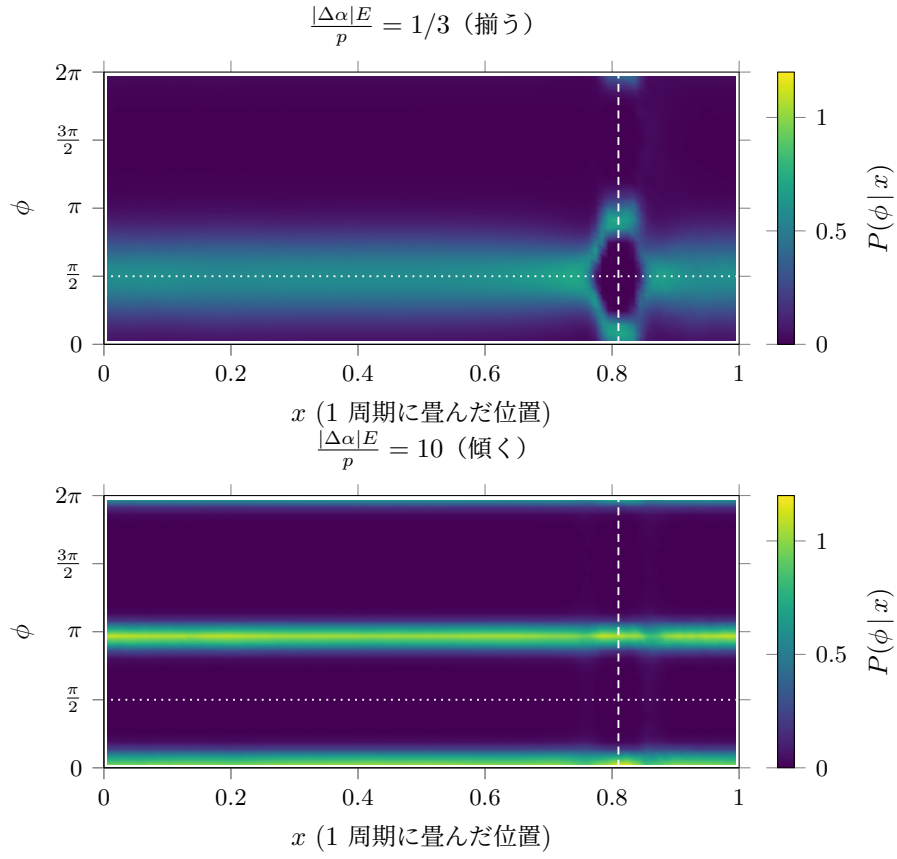
図3 (x, \phi) 占有マップ ( m = 6 , \beta p E = 3 ). 色は各位置 x での条件付き配向分布 P(\phi|x) . 破線は最狭窄部 x \approx 0.81 , 点線は \phi = \pi/2 . \delta = 1/3 (上) では棒は広域で \phi = \pi/2 に揃うが最狭窄部でのみ軸方向に選別され, \delta = 10 (下) では全域で軸方向に傾いて最狭窄部を乱されずに通過する.
