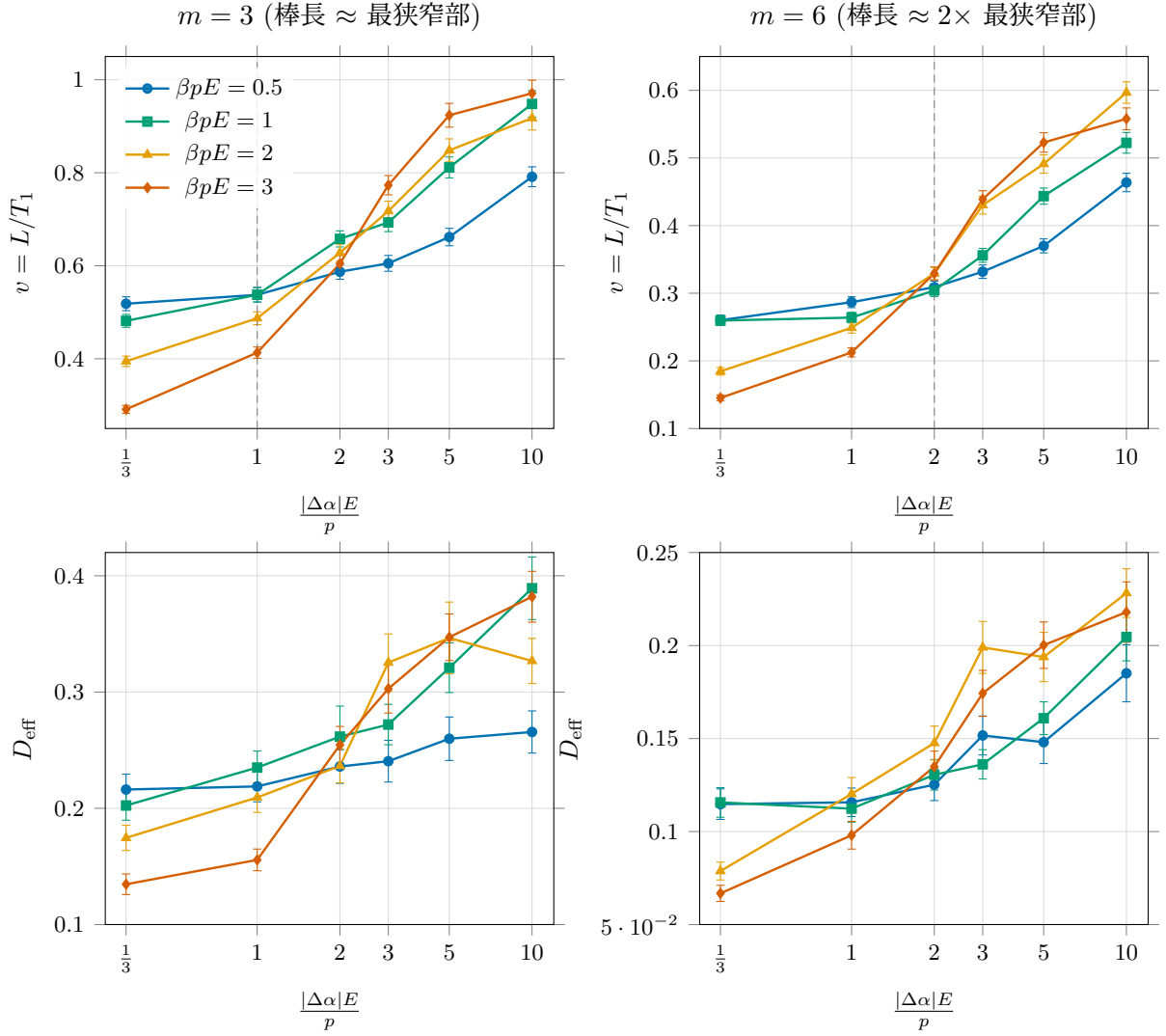
図1 平均速度 v = L/T_1 (上段) と有効拡散係数 D_{\text{eff}} (下段) の \delta = |\Delta\alpha|E/p 依存性. 左列が m = 3 , 右列が m = 6 . 記号は永久双極子と熱エネルギーの比 \beta pE を表す. 誤差棒は初通過時間のブートストラップ標準誤差, 破線は傾いた配向が最狭窄部に収まる幾何閾値 ( m = 3 で \delta = 1 , m = 6 で \delta = 2 ) を示す.
