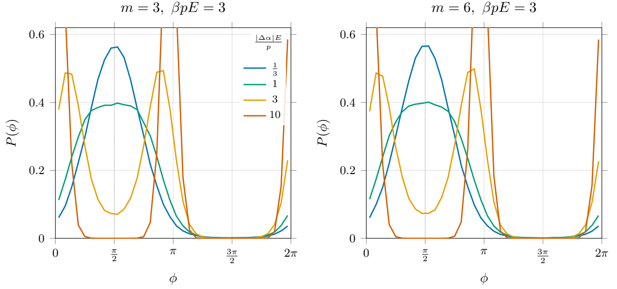
図2 広い断面 ( x \approx 0.20 ) における配向分布 P(\phi) ( m = 3 と m = 6 , いずれも \beta pE = 3 ). \delta が小さいと \phi = \pi/2 (点線) に単峰, 大きいと \phi_1 = \arcsin(1/\delta) 付近 (軸方向) へ移動して二峰化する.
