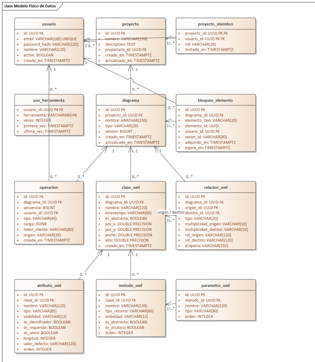
Figura 8. Modelo físico de datos. Cada caja es una tabla con sus columnas y el tipo de PostgreSQL; PK marca la clave primaria —compuesta en proyecto_miembro y en uso_herramienta— y FK la clave ajena. Las flechas son las restricciones referenciales. relacion_uml referencia dos veces a clase_uml, por origen_id y por destino_id, y se dibuja con un solo conector porque ambos van entre las mismas dos cajas.
