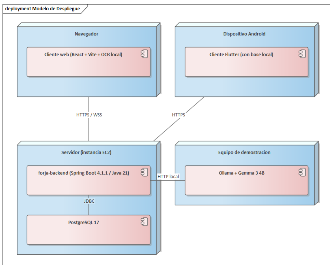
Figura 6. Modelo de despliegue. El equipo de demostración aparece separado porque el modelo de lenguaje no se despliega junto al servidor.
