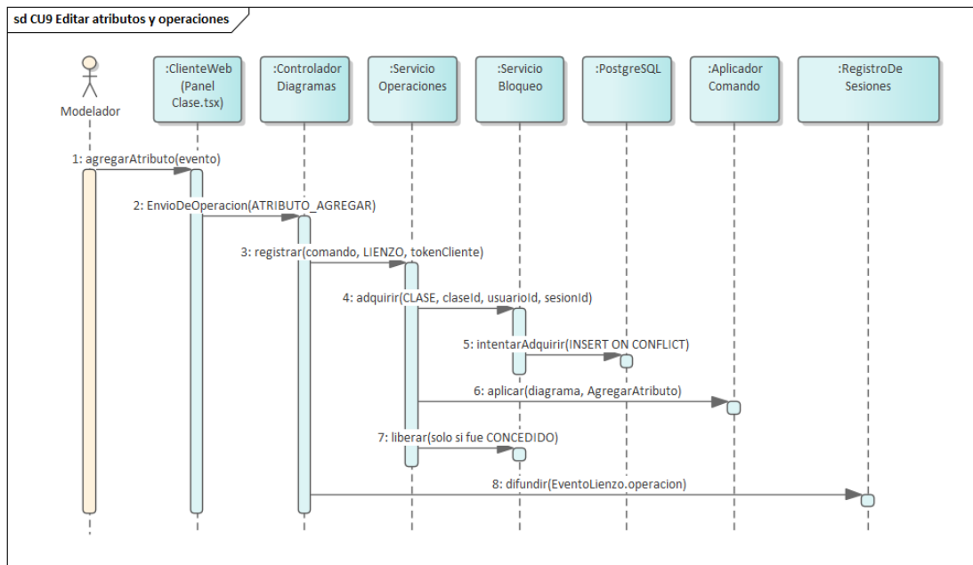
Figura 39. Secuencia — CU9, editar atributos y operaciones. Es donde se ve la exclusión mutua en el camino normal: el bloqueo del paso 4 se pide, no se comprueba, y el 7 solo lo libera si el 4 lo concedió.
