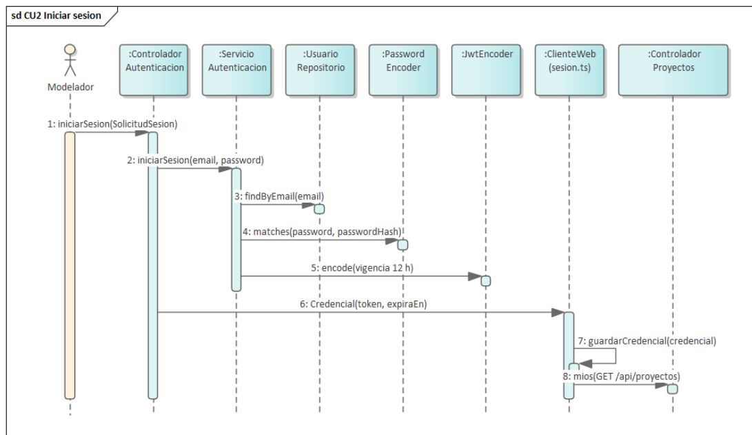
Figura 25. Secuencia — CU2, iniciar sesión. El paso 4 se ejecuta aun sobre una cuenta inactiva, para que el tiempo de respuesta no delate el estado de la cuenta.
