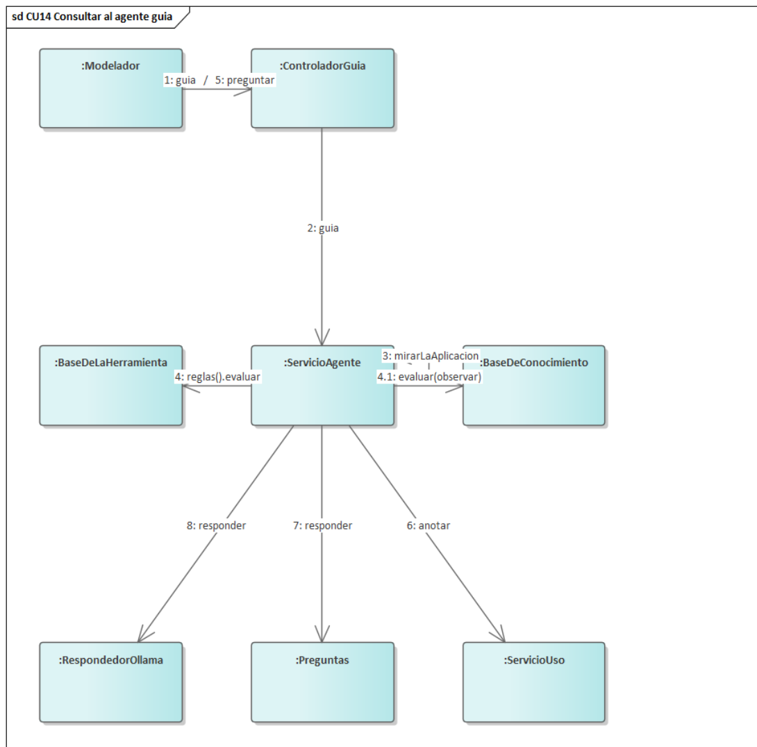
Figura 50. Comunicación — CU14, consultar al agente guía. El modelo del mensaje 8 es el último recurso: solo se le pregunta cuando el catálogo determinista del 7 no engancha. Los rótulos llevan el número y el nombre del mensaje; la firma completa de cada uno está en la tabla que sigue.
