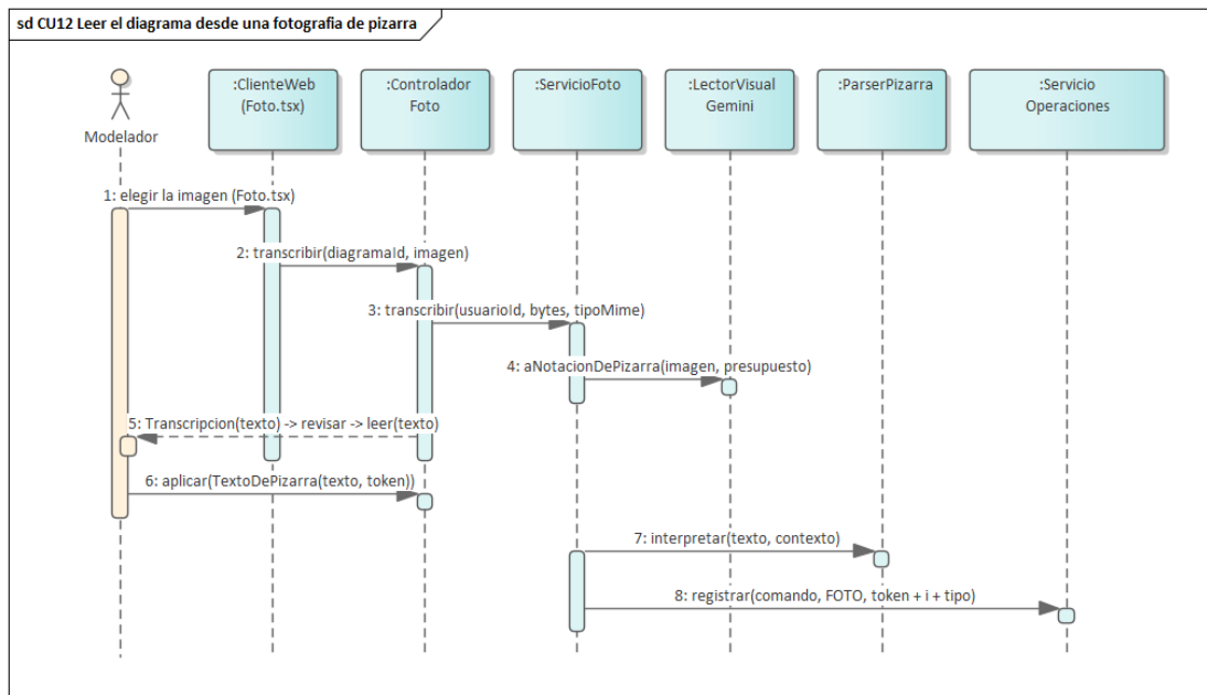
Figura 45. Secuencia — CU12, leer el diagrama desde una fotografía de pizarra. Son tres pasos y no dos: transcribir, leer y aplicar. Entre el 5 y el 6 la persona revisa el texto, y hasta el 6 no se toca el modelo.
