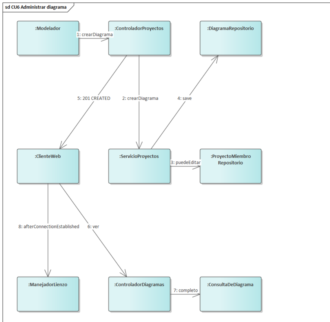
Figura 33. Secuencia — CU6, administrar diagrama. Crear el diagrama y abrirlo son dos peticiones distintas; el paso 8 es la apertura del canal, que registra la sesión en el lienzo.
