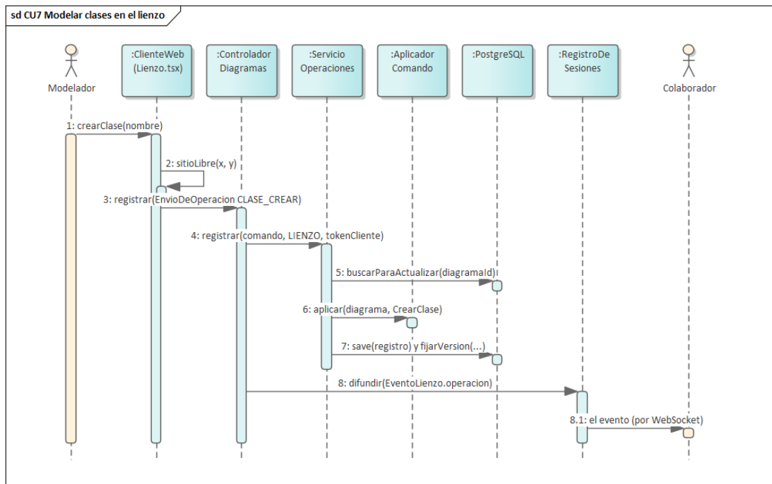
Figura 35. Secuencia — CU7, modelar clases en el lienzo. Es el camino canónico de la herramienta: los mensajes 4 a 7 son los que reutilizan CU11, CU12, CU13, CU17 y CU18. El 8.1 es la segunda mitad del mensaje 8, el evento que el registro de sesiones entrega al colaborador por WebSocket.
