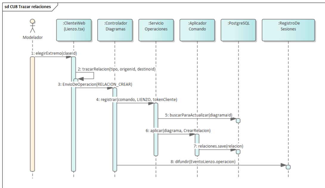
Figura 37. Secuencia — CU8, trazar relaciones. El paso 6 rechaza la herencia y la realización reflexivas, y el 7 pone "1" como multiplicidad por defecto de cada extremo.
