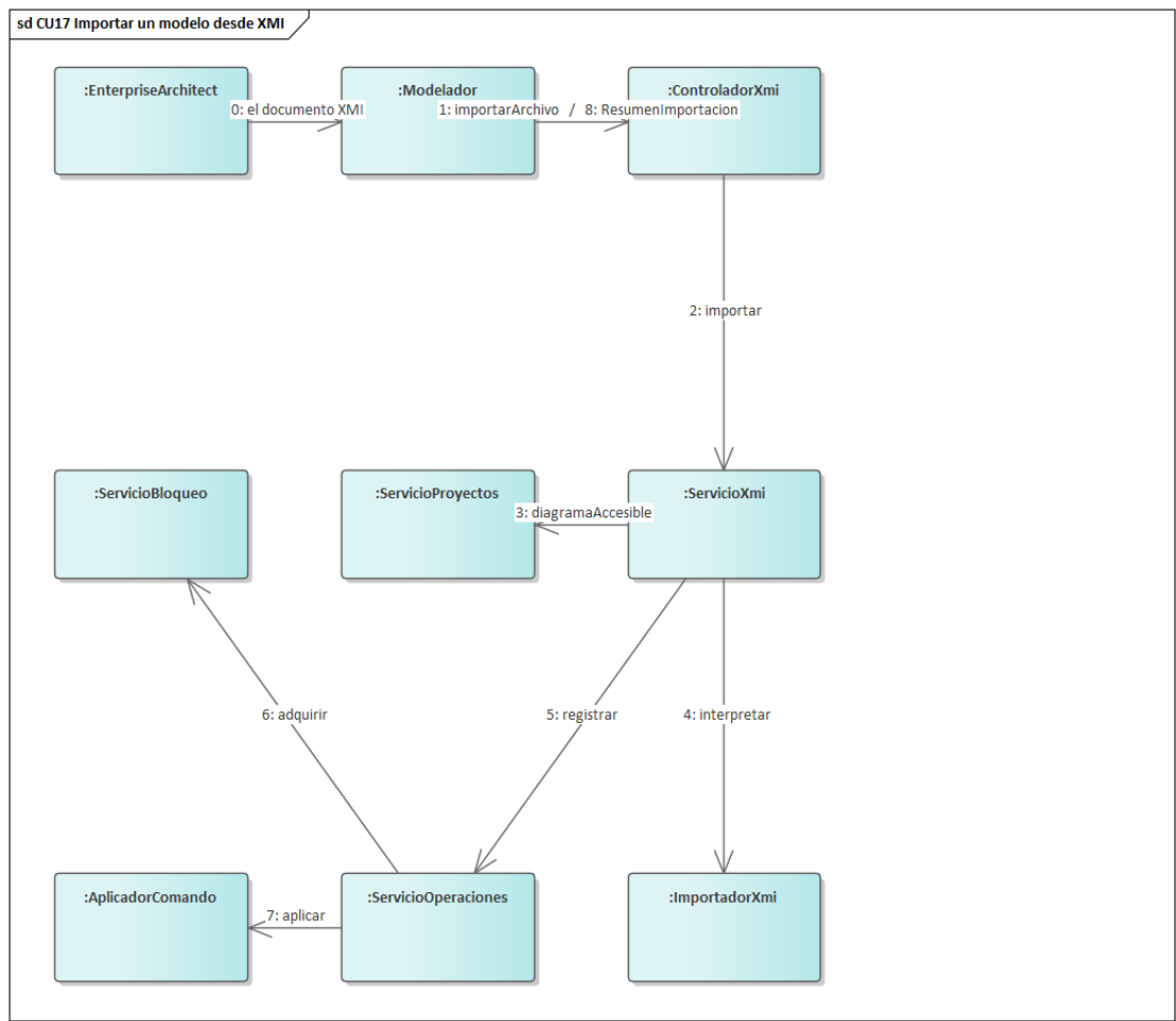
Figura 56. Comunicación — CU17, importar un modelo desde XMI. Importar sobre un diagrama abierto no atropella a quien lo está editando: el bloqueo del mensaje 6 devuelve esos comandos como rechazados. Los rótulos llevan el número y el nombre del mensaje; la firma completa de cada uno está en la tabla que sigue.
