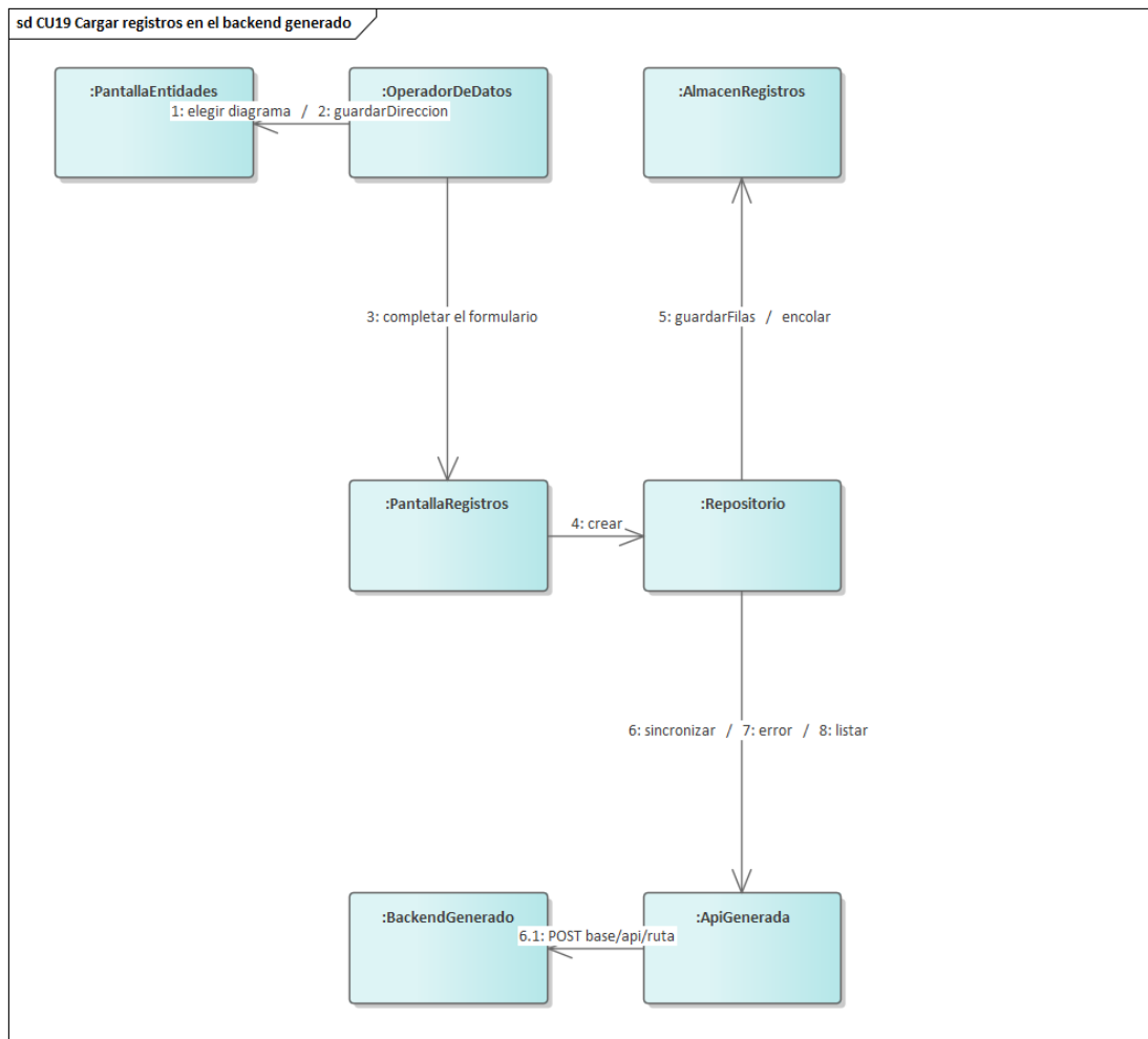
Figura 60. Comunicación — CU19, cargar registros en el backend generado desde el teléfono. Se ve primero y se manda después: el mensaje 5 guarda la fila marcada como pendiente antes de que el 6 la envíe. Los rótulos llevan el número y el nombre del mensaje; la firma completa de cada uno está en la tabla que sigue.
