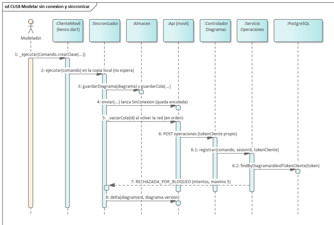
Figura 57. Secuencia — CU18, modelar sin conexión y sincronizar. La pantalla nunca espera al servidor: el paso 2 aplica sobre la copia local. Los mensajes 6.1 y 6.2 son la continuación del 6 dentro del servidor, y el 6.2 es el que evita que un reenvío duplique nada.
