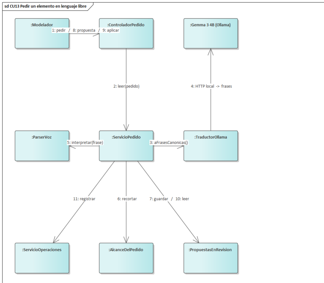
Figura 48. Comunicación — CU13, pedir un elemento en lenguaje libre. Lo que devuelve el modelo pasa siempre por la gramática determinista antes de convertirse en comando, y el alcance lo recorta a un solo elemento antes de mostrarlo. Los rótulos llevan el número y el nombre del mensaje; la firma completa de cada uno está en la tabla que sigue.
