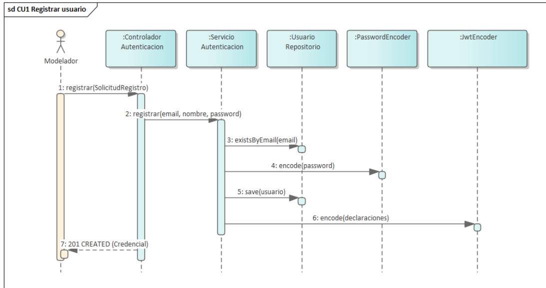
Figura 23. Secuencia — CU1, registrar usuario. La contraseña no se guarda: el paso 4 la reemplaza por su resumen, y el sujeto de la credencial del paso 6 es el identificador y no el correo.
