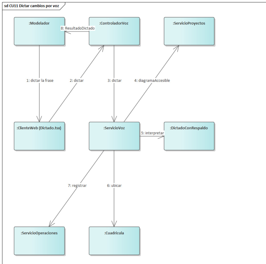
Figura 44. Comunicación — CU11, dictar cambios por voz. La gramática determinista va primero siempre; al modelo local solo se le pide que reescriba la frase cuando ella no entiende. Los rótulos llevan el número y el nombre del mensaje; la firma completa de cada uno está en la tabla que sigue.
