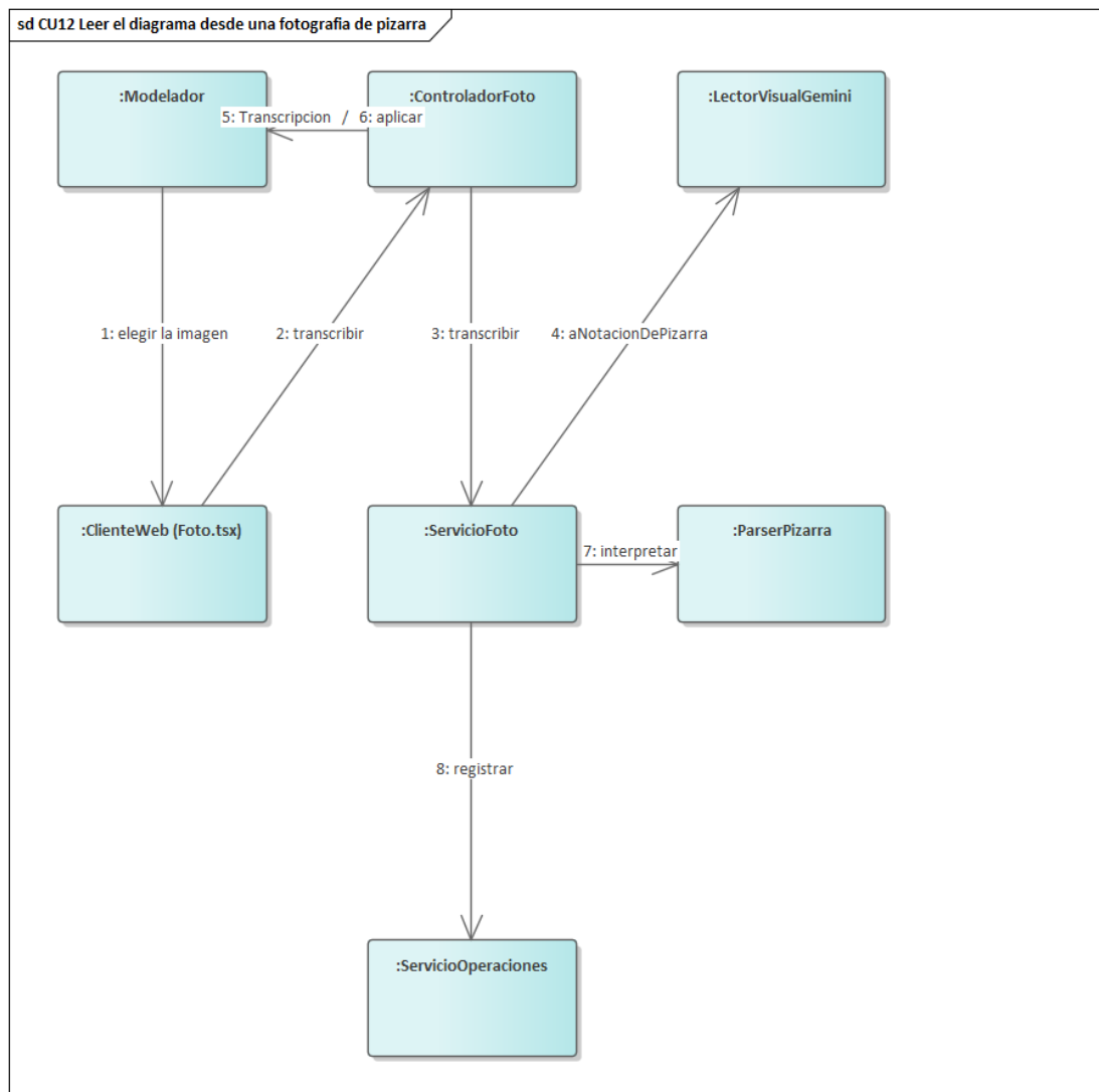
Figura 46. Comunicación — CU12, leer el diagrama desde una fotografía de pizarra. El modelo de visión corre en el servidor porque la clave de pago no puede quedar en el navegador. Los mensajes 5 y 6 comparten enlace. Los rótulos llevan el número y el nombre del mensaje; la firma completa de cada uno está en la tabla que sigue.
