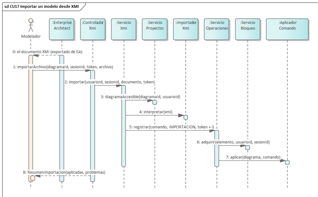
Figura 55. Secuencia — CU17, importar un modelo desde XMI. El mensaje 0 es la precondición: el documento viene de Enterprise Architect. Cada comando se registra en
