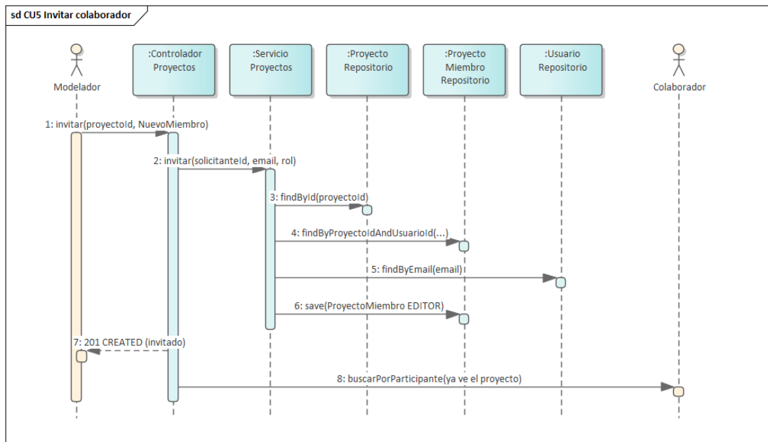
Figura 31. Secuencia — CU5, invitar colaborador. El paso 4 es el que decide: si el rol del solicitante no es propietario, la invitación se rechaza antes de tocar nada.
