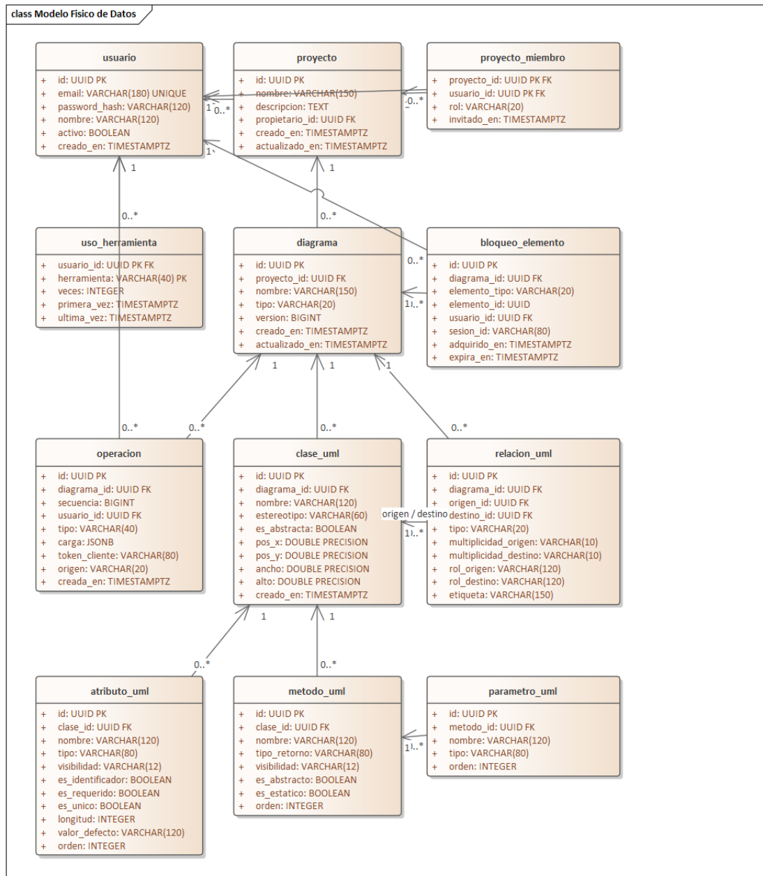
Figura 63. Modelo físico de datos. Cada caja es una tabla con sus columnas y el tipo de PostgreSQL; PK marca la clave primaria —compuesta en proyecto_miembro y en uso_herramienta — y FK la clave ajena. Las flechas son las restricciones referenciales. relacion_uml referencia dos veces a clase_uml , por origen_id y por destino_id , y se dibuja con un solo conector porque ambos van entre las mismas dos cajas.
