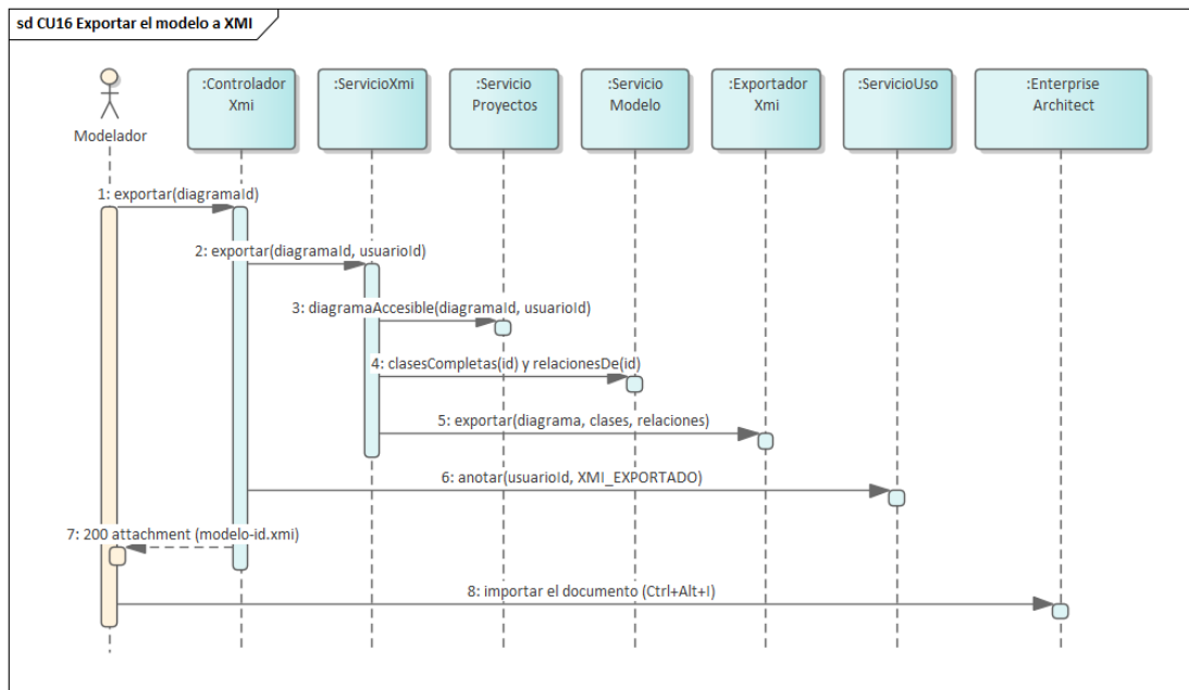
Figura 53. Secuencia — CU16, exportar el modelo a XMI. La disposición de cada clase viaja en el bloque de extensión de Enterprise Architect, y el documento se importa en EA, no se abre.
