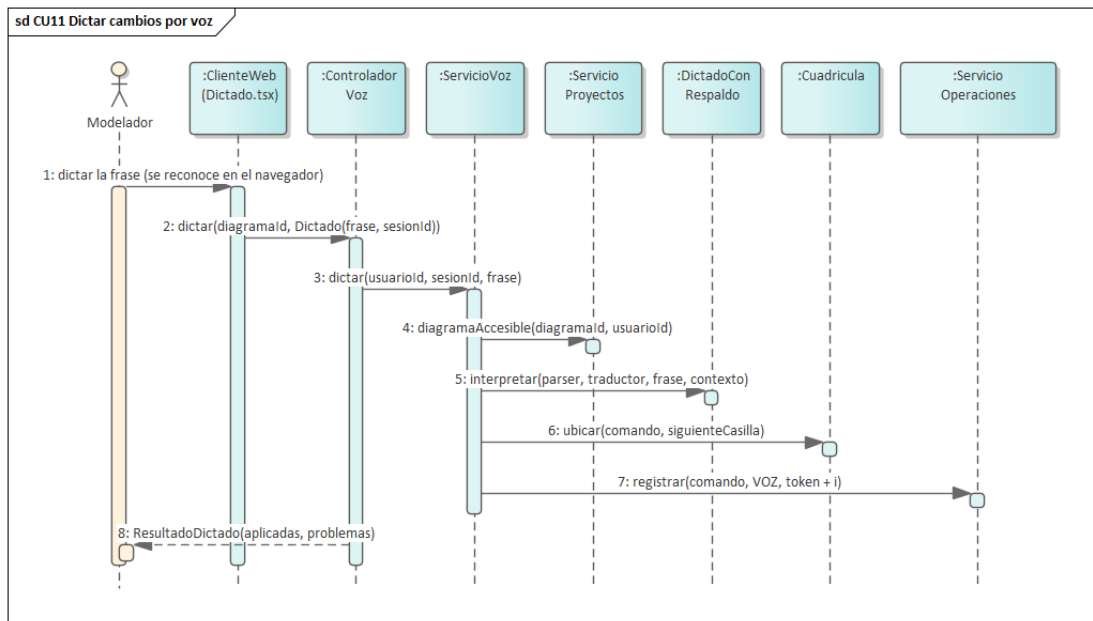
Figura 43. Secuencia — CU11, dictar cambios por voz. El reconocimiento de voz ocurre en el navegador: lo que sube al servidor es texto. El paso 7 es el mismo punto de entrada de CU7, CU8 y CU9.
