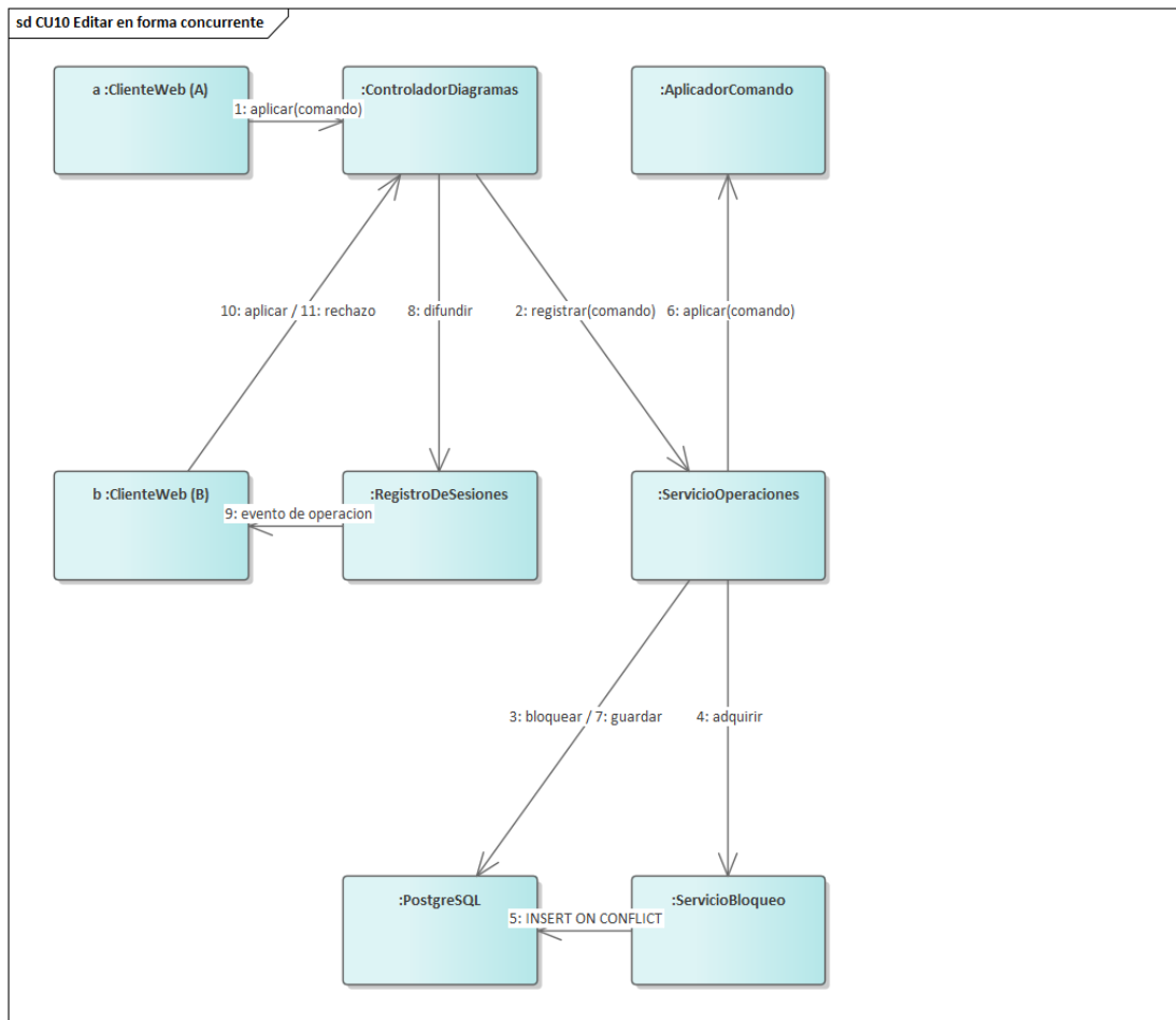
Figura 42. Comunicación — CU10, editar en forma concurrente. Los objetos son las clases reales del servidor; a y b son los clientes web de la persona A y de la persona B. La persona B intenta el mismo elemento que la persona A y es rechazada en el paso 11. Los rótulos llevan el número y el nombre del mensaje; la firma completa de cada uno está en la tabla que sigue.
