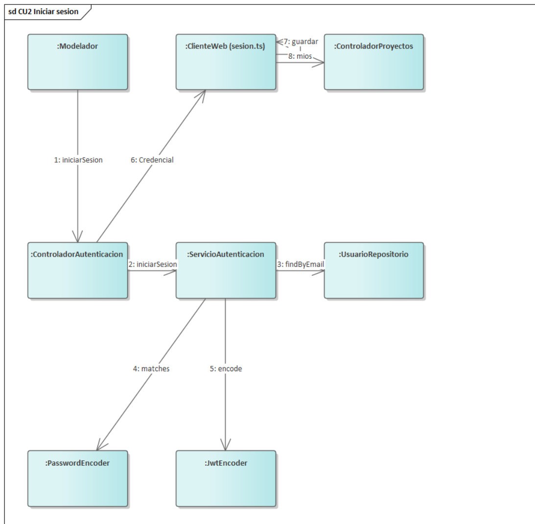
Figura 26. Comunicación — CU2, iniciar sesión. El mensaje 7 es el único que un objeto se manda a sí mismo: guardar la credencial es trabajo del navegador. Los rótulos llevan el número y el nombre del mensaje; la firma completa de cada uno está en la tabla que sigue.
