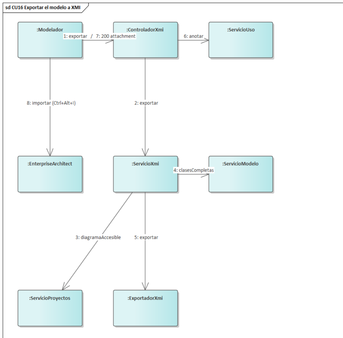
Figura 54. Comunicación — CU16, exportar el modelo a XMI. Enterprise Architect es el destinatario del documento y el único participante que no es parte de FORJA. Los rótulos llevan el número y el nombre del mensaje; la firma completa de cada uno está en la tabla que sigue.
