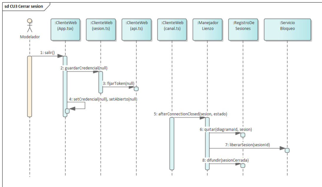
Figura 27. Secuencia — CU3, cerrar sesión. No hay petición de cierre de sesión: el token no tiene estado en el servidor y cerrarla es tirarlo. Lo único que llega al servidor es el cierre del WebSocket, del paso 5 en adelante, que es lo que devuelve los bloqueos.
