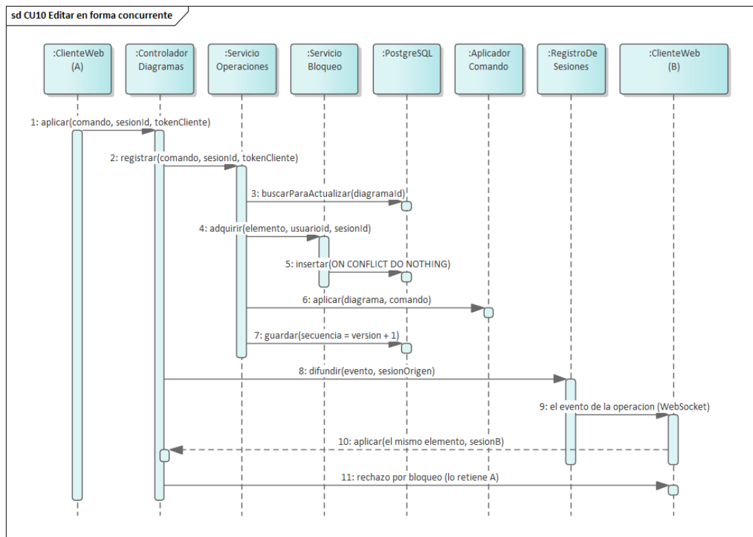
Figura 41. Secuencia — CU10, editar en forma concurrente. La persona B intenta el mismo elemento que la persona A mientras esta lo retiene, y es rechazada en el paso 11.
