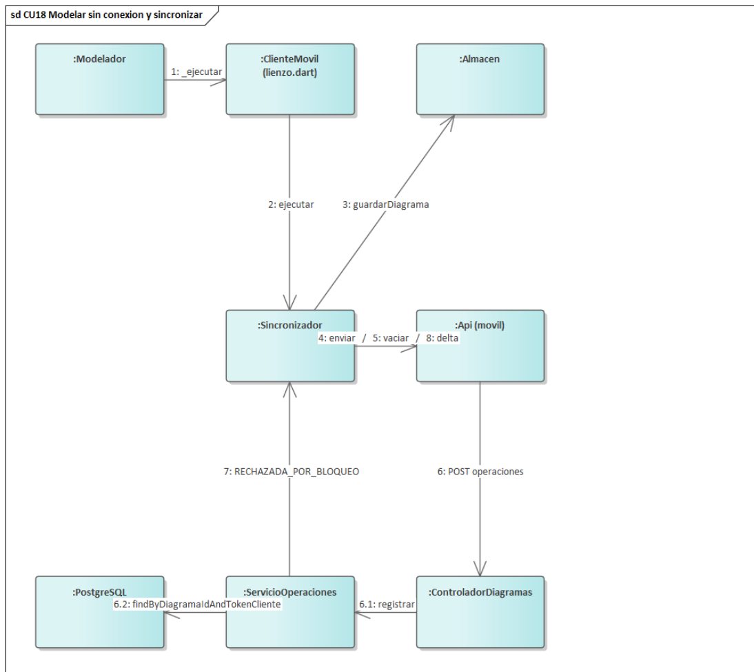
Figura 58. Comunicación — CU18, modelar sin conexión y sincronizar. El delta del mensaje 8 se pide solo después de vaciar la cola: al revés traería un estado que todavía no incluye lo propio. Los rótulos llevan el número y el nombre del mensaje; la firma completa de cada uno está en la tabla que sigue.
