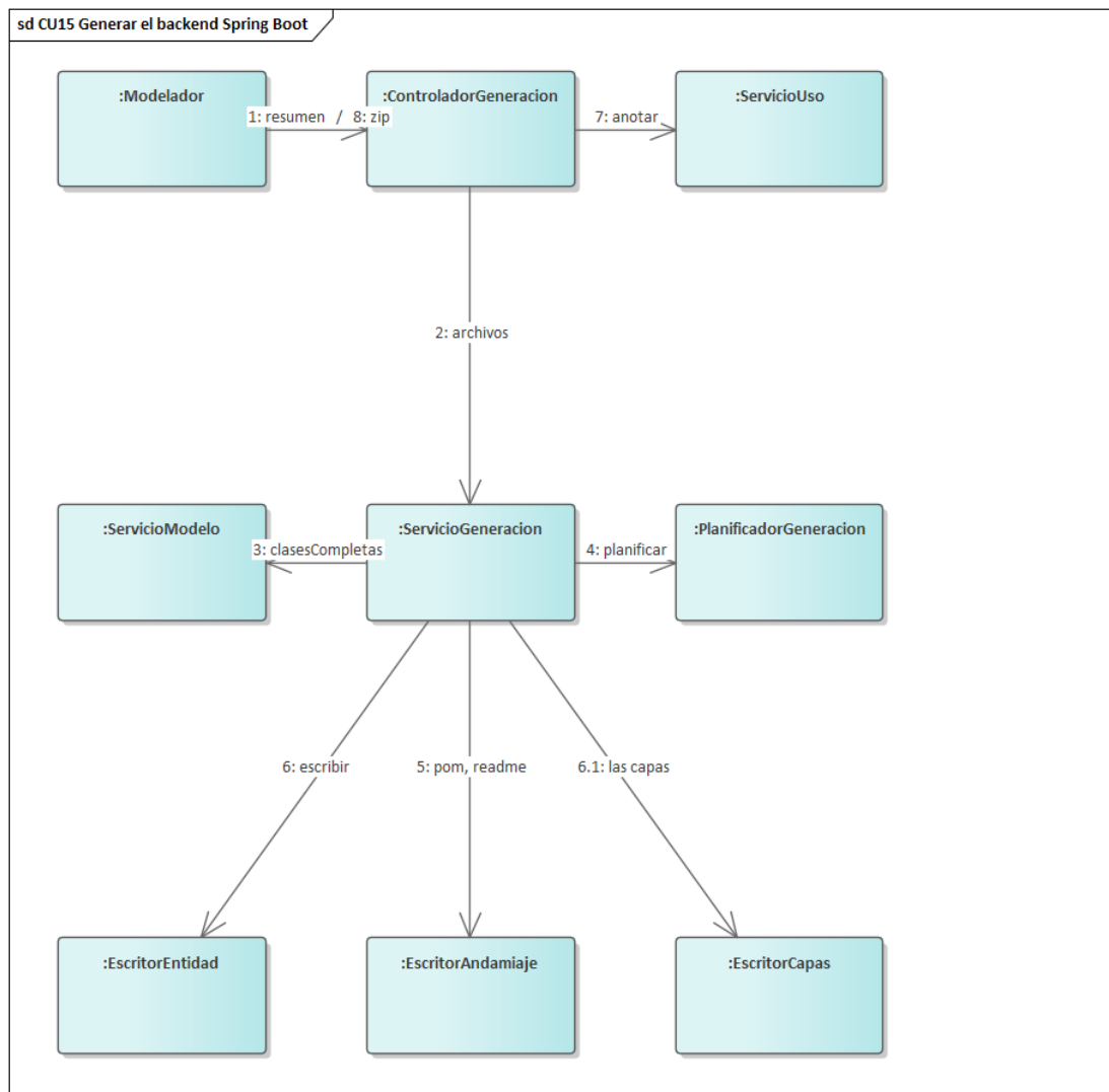
Figura 52. Comunicación — CU15, generar el backend Spring Boot. Generar no cambia el modelo, así que no entra en la bitácora de operaciones: lo único que queda anotado es el uso, en el mensaje 7. Los rótulos llevan el número y el nombre del mensaje; la firma completa de cada uno está en la tabla que sigue.
