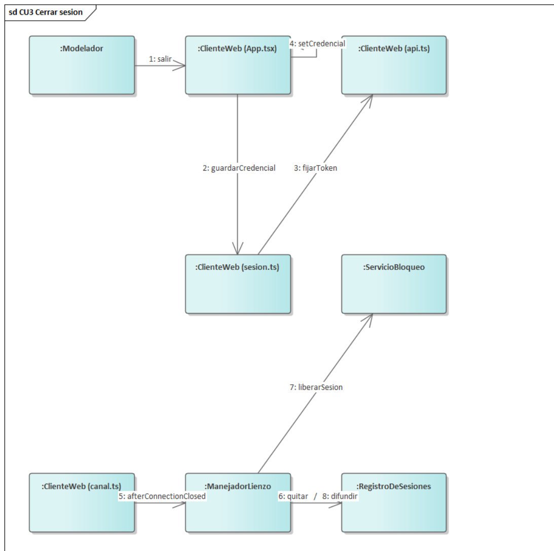
Figura 28. Comunicación — CU3, cerrar sesión. Se ven las dos mitades del caso, que no se comunican entre sí: la del navegador y la que dispara el cierre del canal. Los rótulos llevan el número y el nombre del mensaje; la firma completa de cada uno está en la tabla que sigue.
