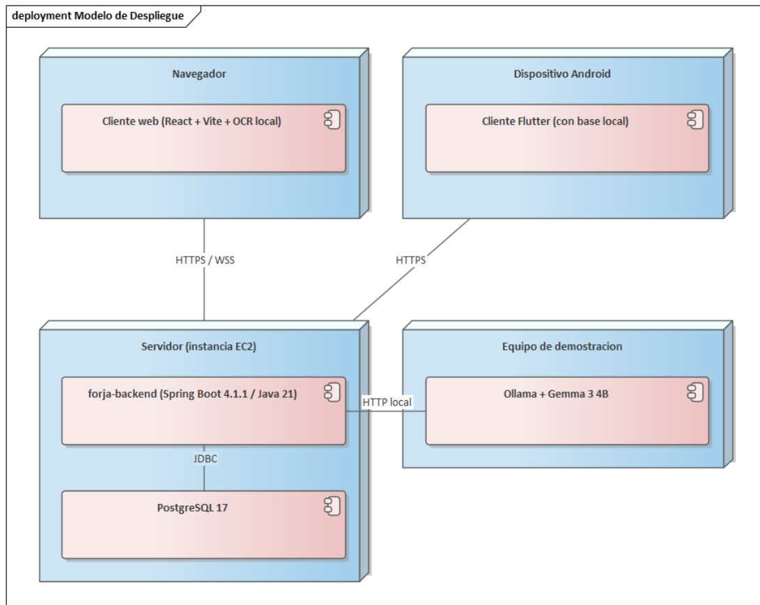
Figura 61. Modelo de despliegue. El equipo de demostración aparece separado porque el modelo de lenguaje no se despliega junto al servidor.
