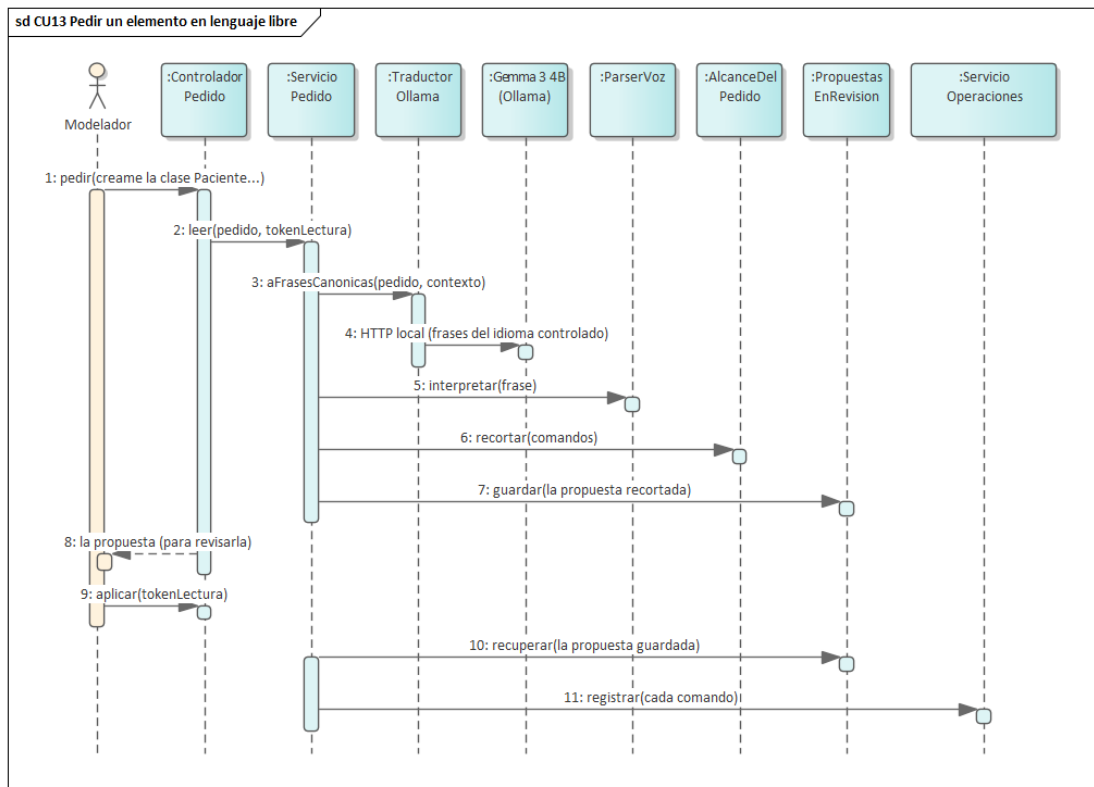
Figura 47. Secuencia — CU13, pedir un elemento en lenguaje libre. El paso 10 recupera la propuesta guardada en vez de volver a consultar al modelo: es lo que hace que lo aplicado sea lo revisado.
