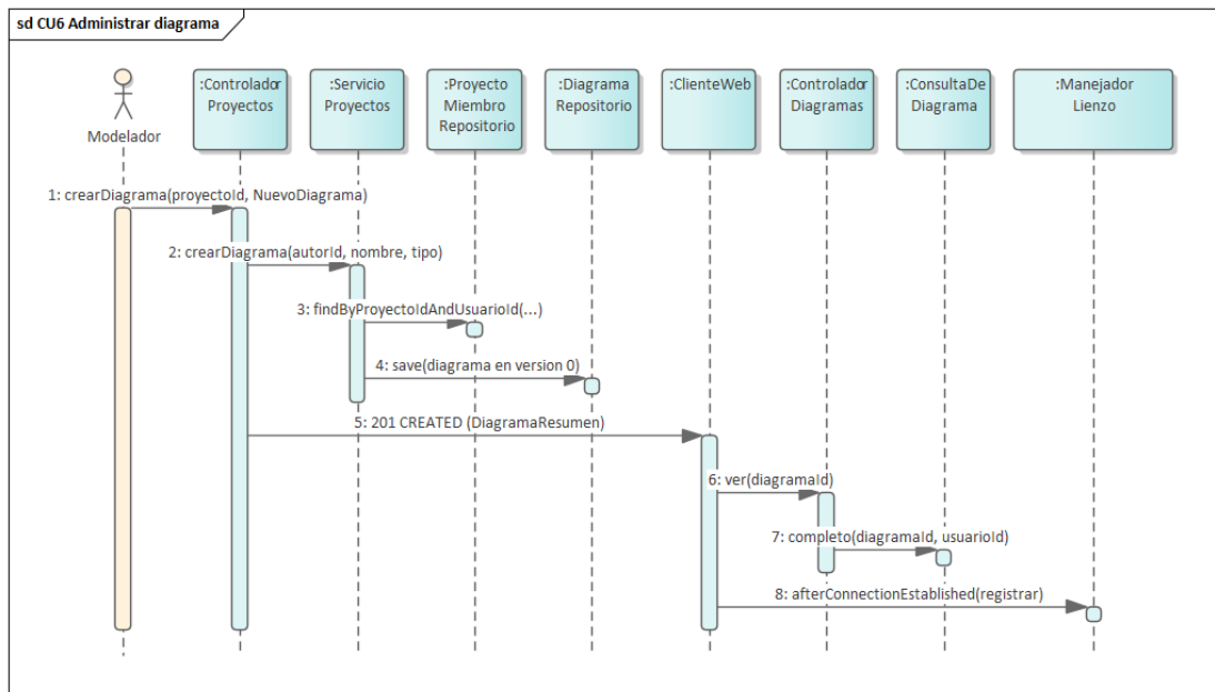
Figura 33. Secuencia — CU6, administrar diagrama. Crear el diagrama y abrirlo son dos peticiones distintas; el paso 8 es la apertura del canal, que registra la sesión en el lienzo.
