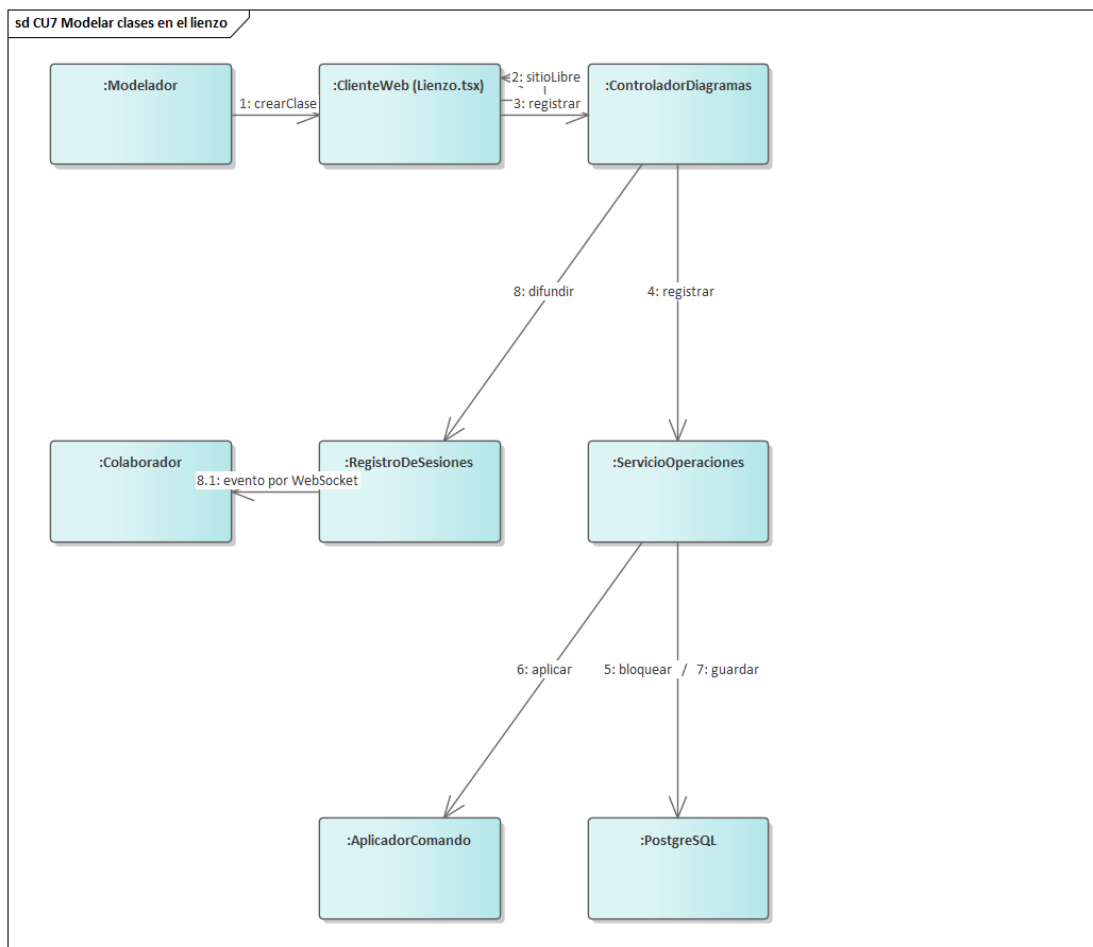
Figura 35. Secuencia — CU7, modelar clases en el lienzo. Es el camino canónico de la herramienta: los mensajes 4 a 7 son los que reutilizan CU11, CU12, CU13, CU17 y CU18. El 8.1 es la segunda mitad del mensaje 8, el evento que el registro de sesiones entrega al colaborador por WebSocket.
