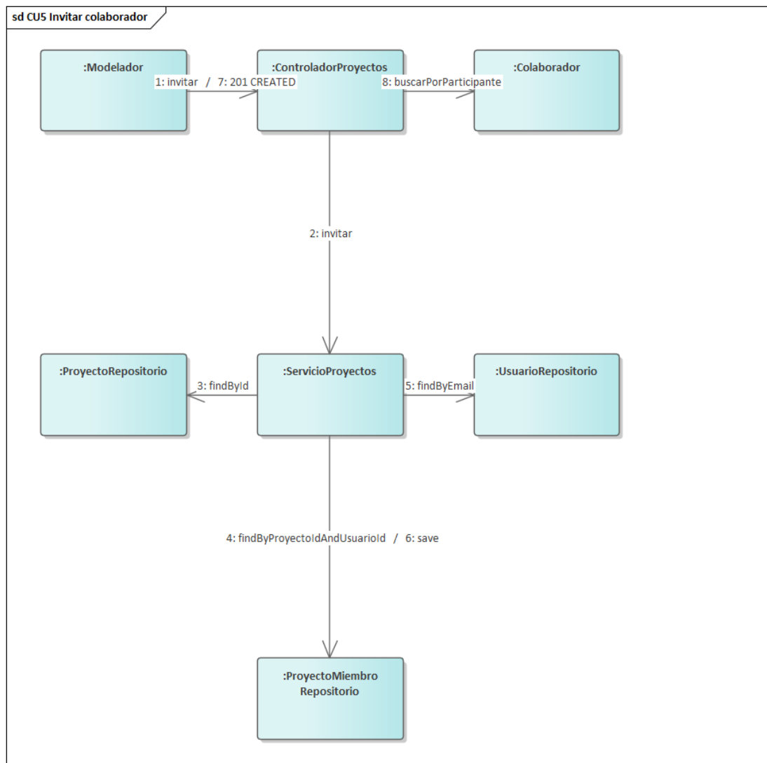
Figura 31. Secuencia — CU5, invitar colaborador. El paso 4 es el que decide: si el rol del solicitante no es propietario, la invitación se rechaza antes de tocar nada.
