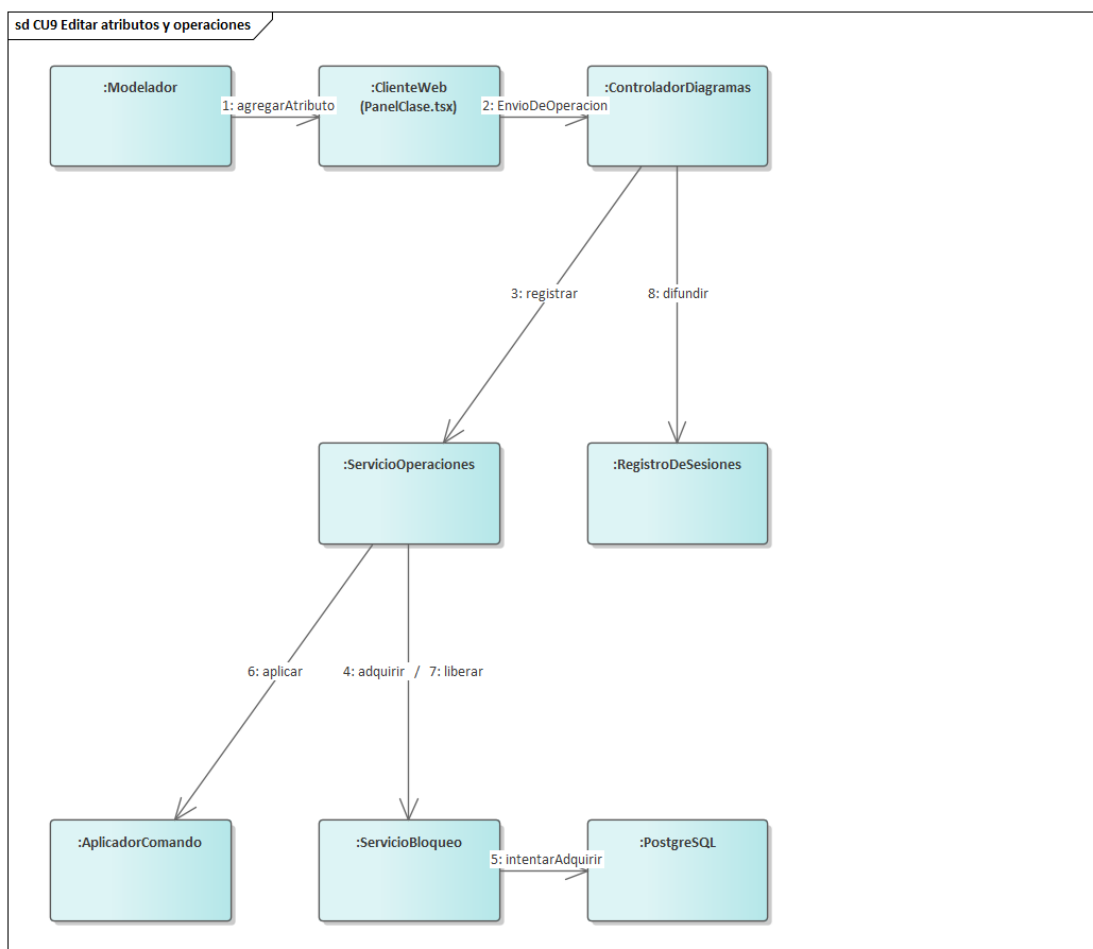
Figura 40. Comunicación — CU9, editar atributos y operaciones. Los mensajes 4 y 7 comparten enlace: son la toma y la devolución del mismo bloqueo. Los rótulos llevan el
