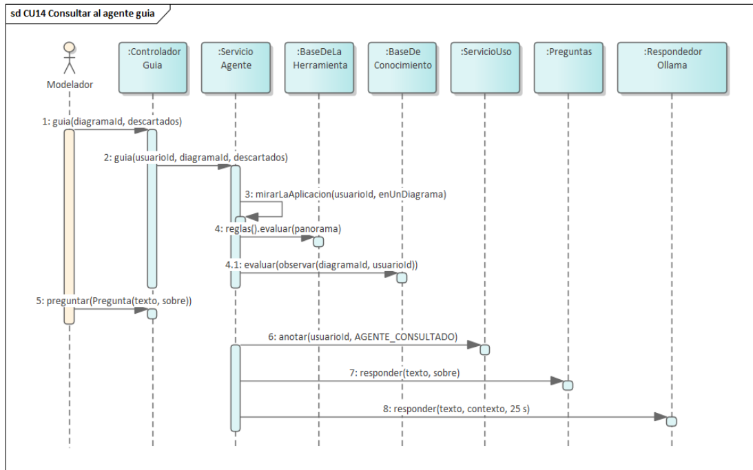
Figura 49. Secuencia — CU14, consultar al agente guía. Único caso que llega al modelo de lenguaje sin incluir a CU7, CU8 ni CU9: el agente informa, no modifica el diagrama. El 4.1 es la segunda evaluación del mensaje 4, la que solo ocurre cuando hay un diagrama abierto.
