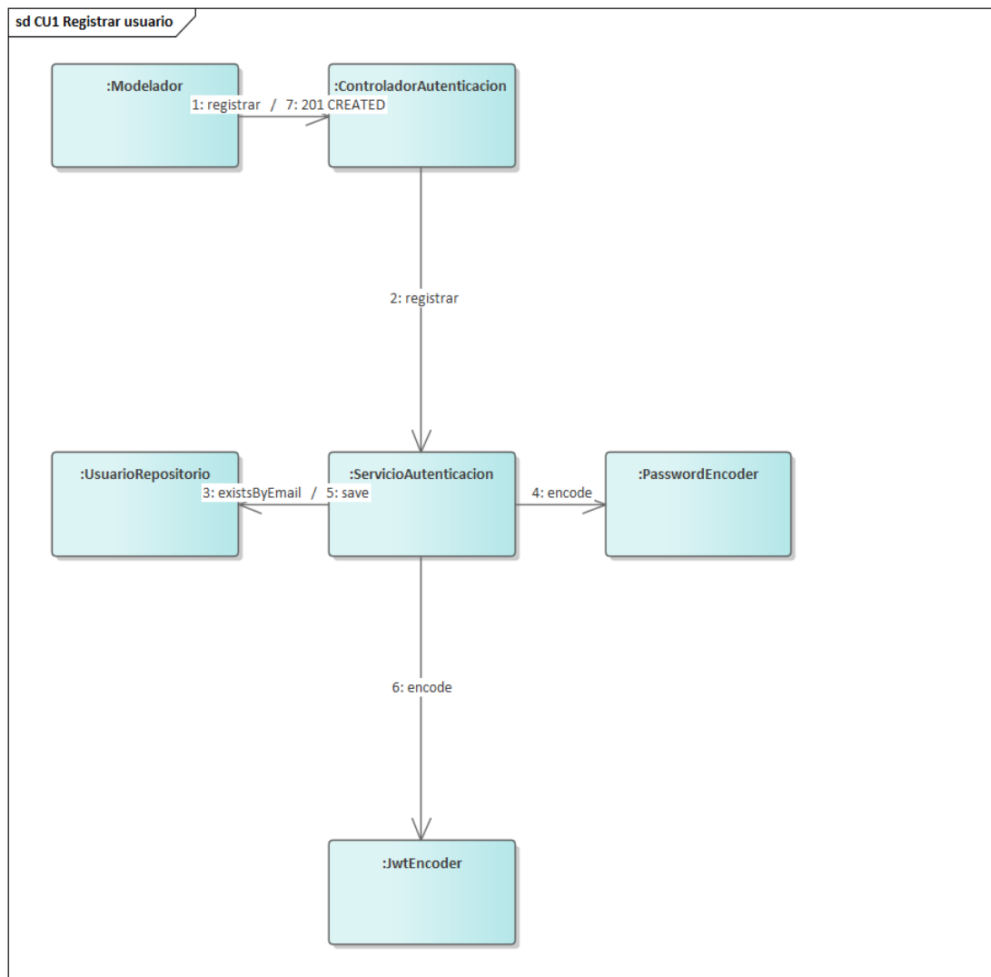
Figura 24. Comunicación — CU1, registrar usuario. Los mensajes 3 y 5 comparten enlace porque viajan entre el mismo par de objetos, y lo mismo el 1 y el 7. Los rótulos llevan el número y el nombre del mensaje; la firma completa de cada uno está en la tabla que sigue.
