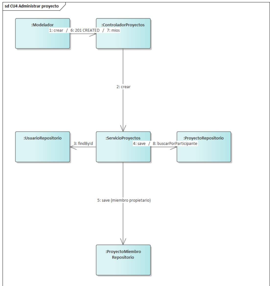
Figura 30. Comunicación — CU4, administrar proyecto. Los mensajes 1, 6 y 7 comparten el enlace con el modelador, y el 4 y el 8 el del repositorio de proyectos. Los rótulos llevan el número y el nombre del mensaje; la firma completa de cada uno está en la tabla que sigue.
