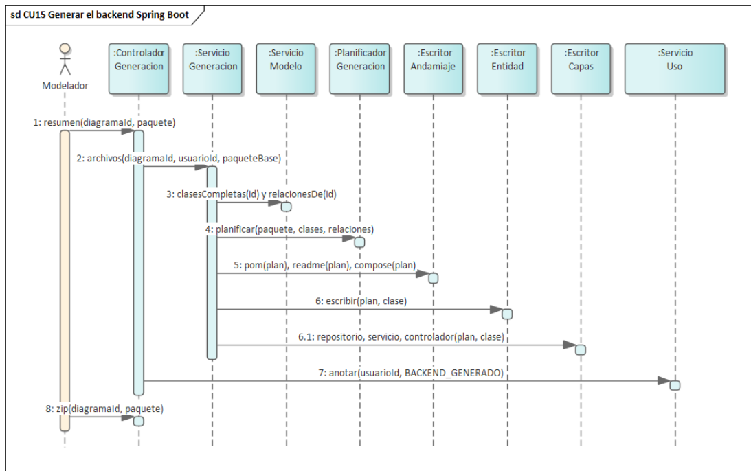
Figura 51. Secuencia — CU15, generar el backend Spring Boot. El paso 4 arma un plan intermedio y los pasos 5, 6 y 6.1 escriben desde ese plan; el 6.1 es la parte del mensaje 6 que produce las otras tres capas.
