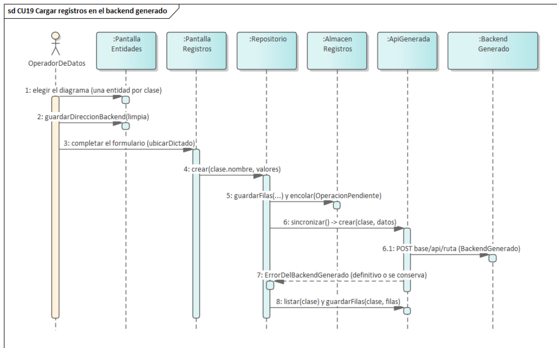
Figura 59. Secuencia — CU19, cargar registros en el backend generado desde el teléfono. Único caso que no toca FORJA: el cliente habla con el backend que la propia herramienta escribió, que es otro sistema y no tiene autenticación. El 6.1 es la petición que la capa de red hace contra él.
