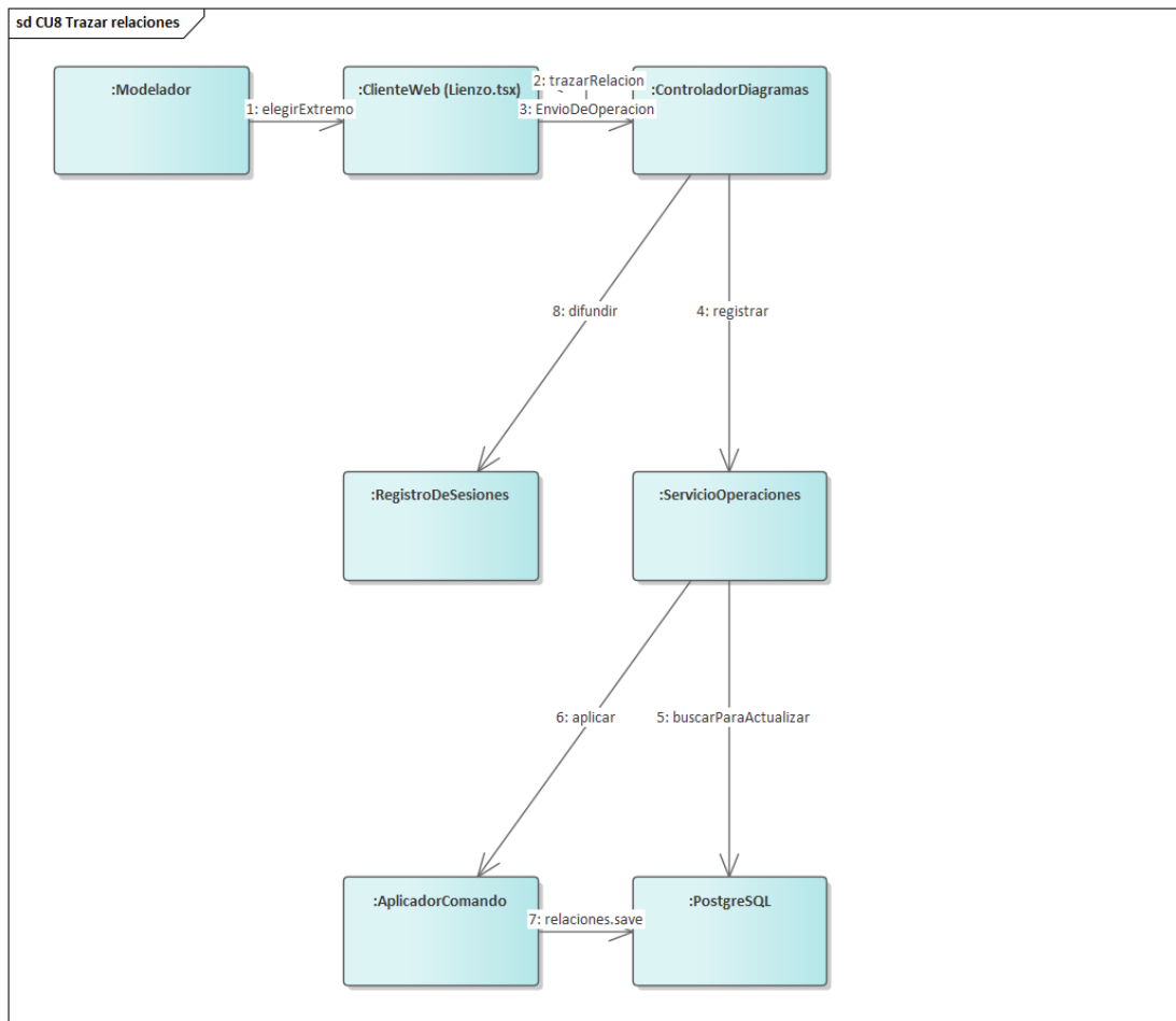
Figura 38. Comunicación — CU8, trazar relaciones. Mismo recorrido que CU7, con una diferencia: aquí es el aplicador, y no el servicio, quien escribe la relación. Los rótulos llevan el número y el nombre del mensaje; la firma completa de cada uno está en la tabla que sigue.
