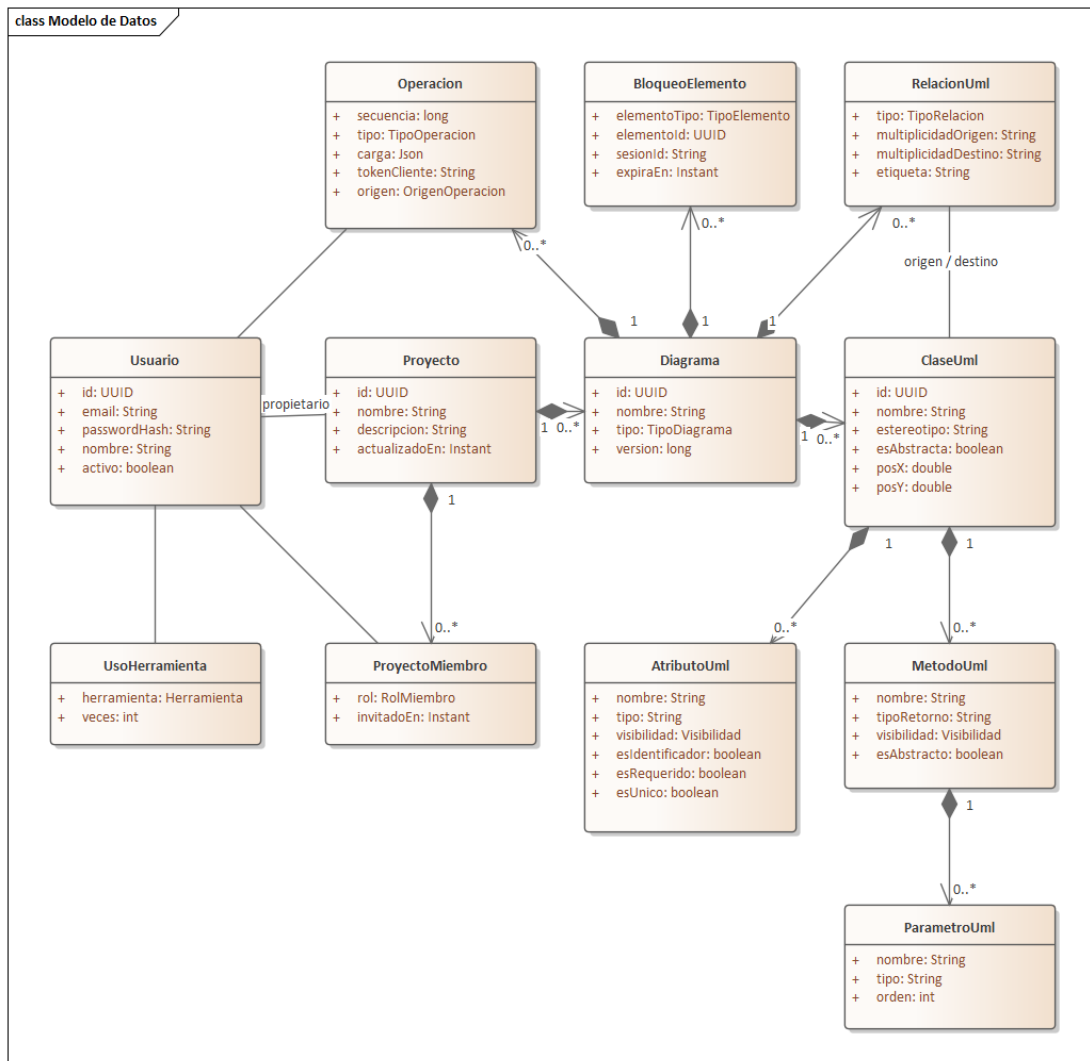
Figura 26. Modelo de datos. La fila del medio es el recorrido del dominio y se lee de izquierda a derecha —Usuario → Proyecto → Diagrama → ClaseUml—; arriba y abajo cuelga lo que se apoya en cada uno. Los rombos rellenos son composiciones: la parte no existe sin el todo, y el esquema lo impone con borrado en cascada.
