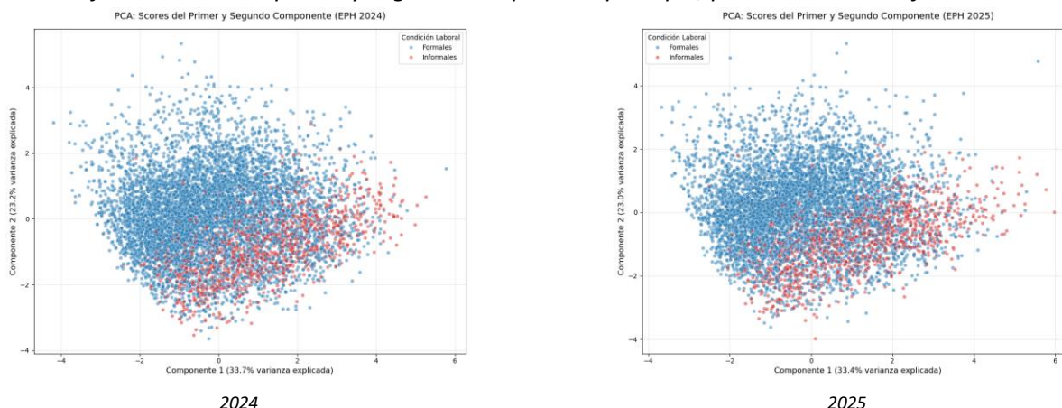
Gráfico 2. Scores del primer y segundo componente principal, por condición de informalidad
