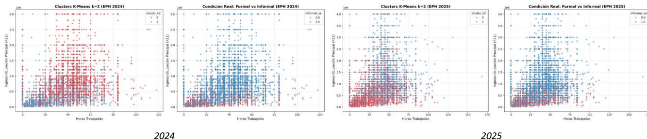
Gráfico 5. Clusters K-medias ( k=2 ) vs. condición real de informalidad – EPH 2024 y 2025
