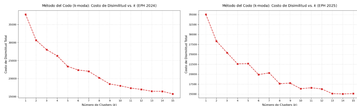
Gráfico 8. Método del Codo ( k -moda) – EPH 2024 y 2025
