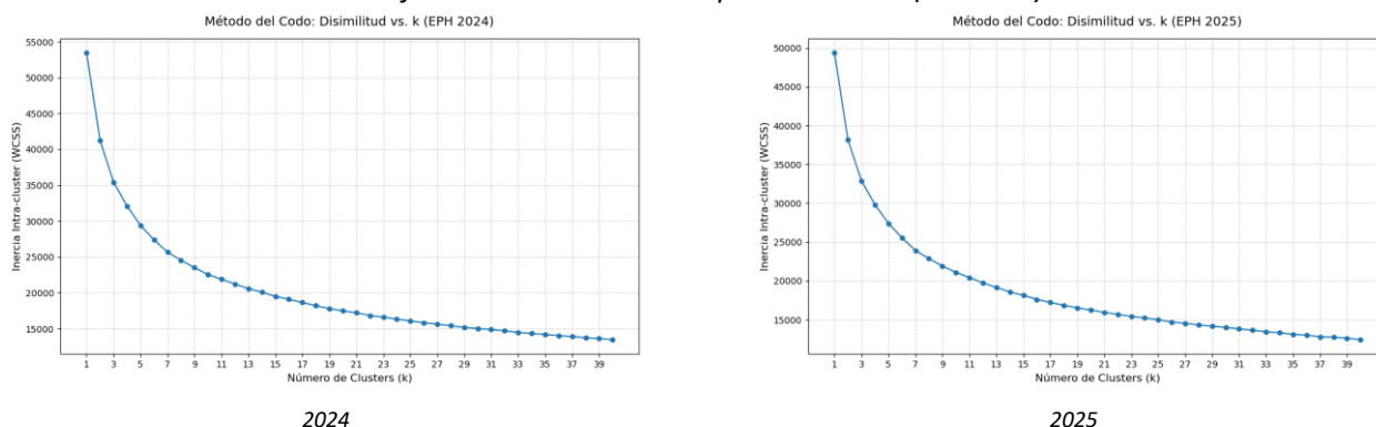
Gráfico 6. Método del codo para k-medias ( k=1 a 40)
