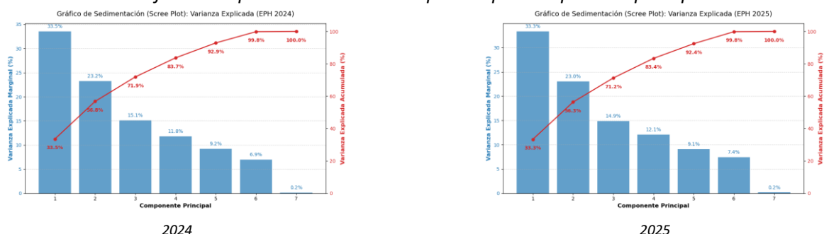
Gráfico 4. Proporción de varianza explicada por componente principal
