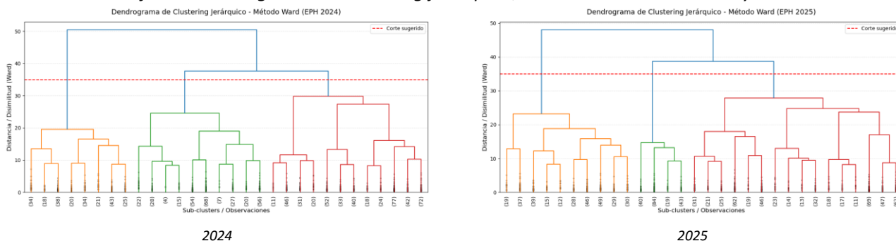
Gráfico 7. Dendrograma de clustering jerárquico, método Ward – EPH 2024 y 2025
