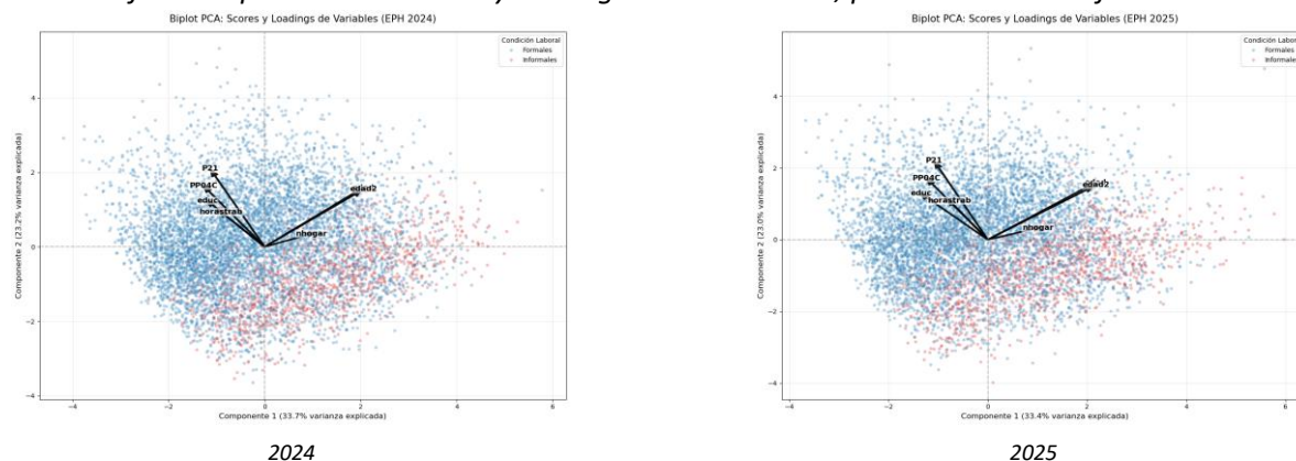
Gráfico 3. Biplot de PCA: scores y loadings de las variables, por condición de informalidad
