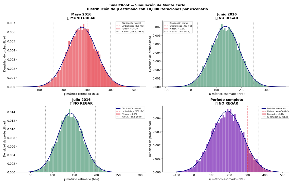
Figura 3: Distribuciones simuladas por Montecarlo (10 000 iteraciones) para los cuatro escenarios. La línea roja punteada indica el umbral de riesgo urgente (300 hPa). El área sombreada rosa representa P(\Psi > 300) .
