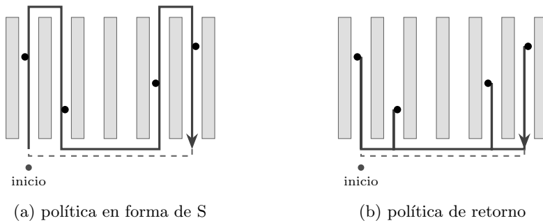
Figura 2.4: Dos políticas de ruteo sobre el mismo layout, con las estanterías en gris y las mismas cuatro extracciones (puntos). La política en S recorre completos solo los pasillos con extracciones, mientras que la de retorno entra y sale de cada uno por el corredor frontal. La línea punteada es la vuelta al inicio.
