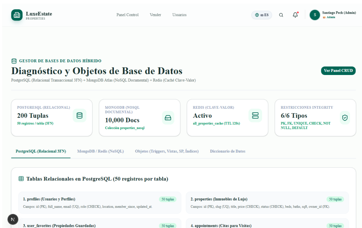
Figura 4. Panel Administrativo de Diagnóstico BD (/admin/database) mostrando objetos de base de datos y diccionario.
