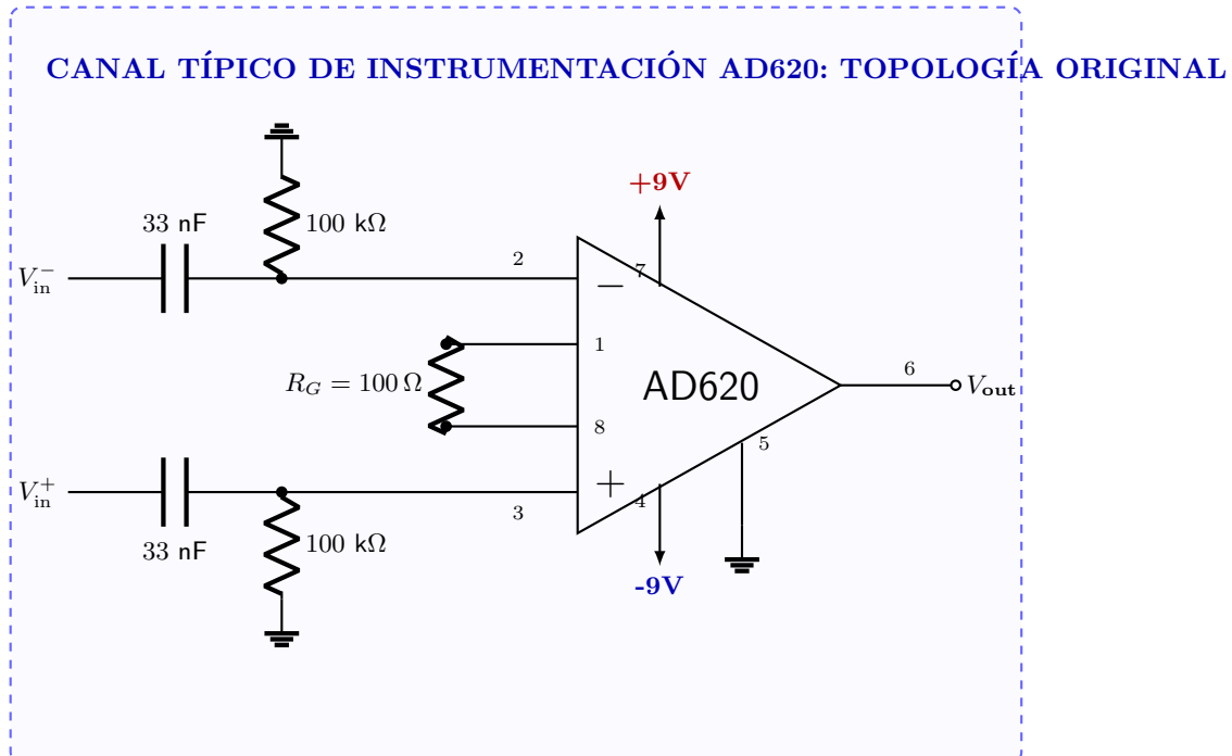
Figura 4: Canal típico de instrumentación diferencial AD620 en su topología original (idéntico para los 3 canales de la placa). Dispone de un filtro pasa-altos pasivo unipolar a la entrada ( C = 33\text{ nF} , R = 100\text{ k}\Omega , f_c \approx 48,23\text{ Hz} ) y resistencia de ganancia fija soldada en placa R_G = 100\text{ }\Omega ( G \approx 495\text{ V/V} ).
