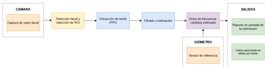
Figura 1. Diagrama en bloques del sistema.
