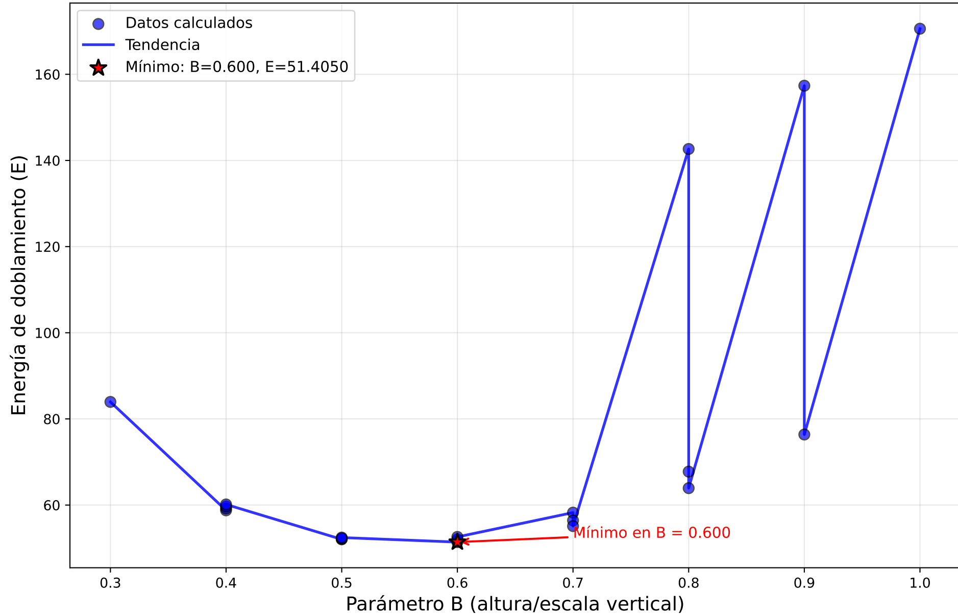
Energía de curvatura vs. Parámetro B (A = 4.60)
