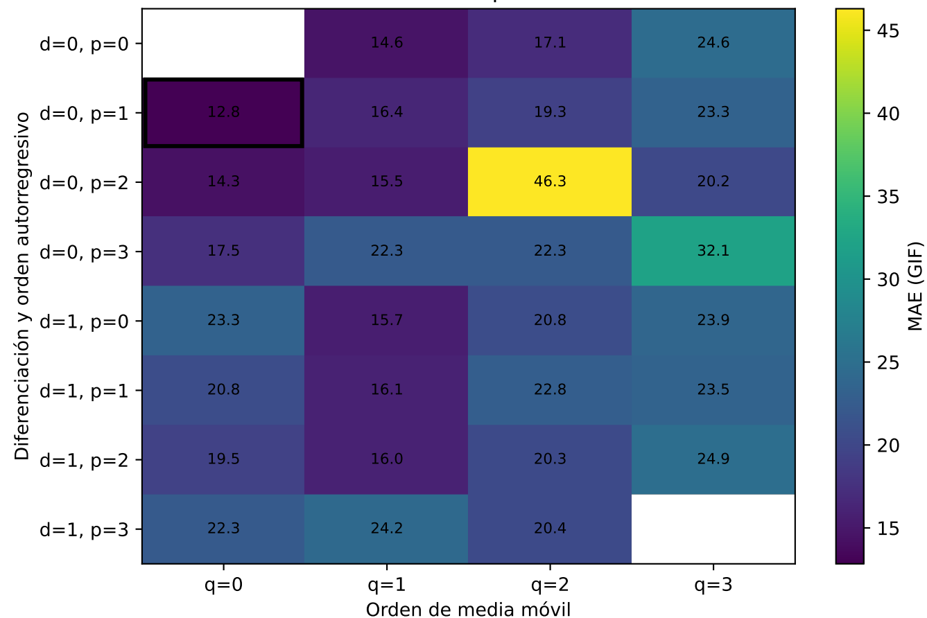
MAE rodante de las 30 especificaciones ARIMA
