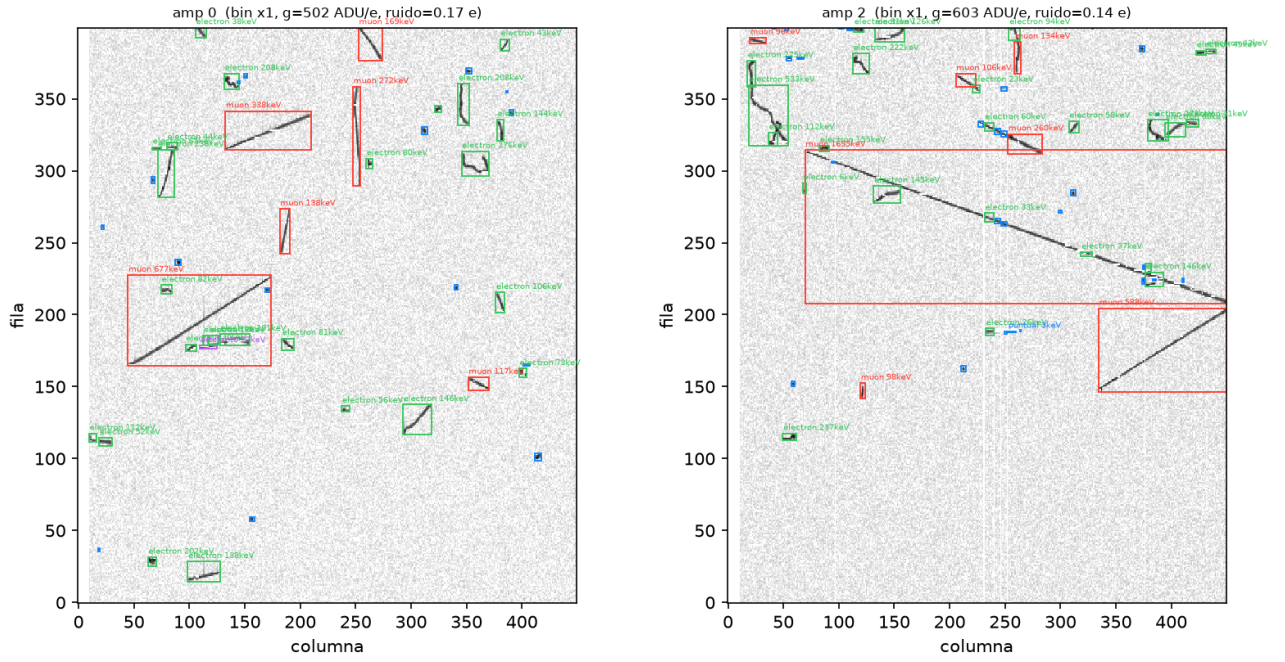
Figura 1: Detecciones por reglas físicas en los amplificadores 0 y 2 de una imagen de Skipper-CCD: muones (rojo), electrones (verde), trazas puntuales (azul) y artefactos (violeta). Las etiquetas indican la energía reconstruida de cada traza.
