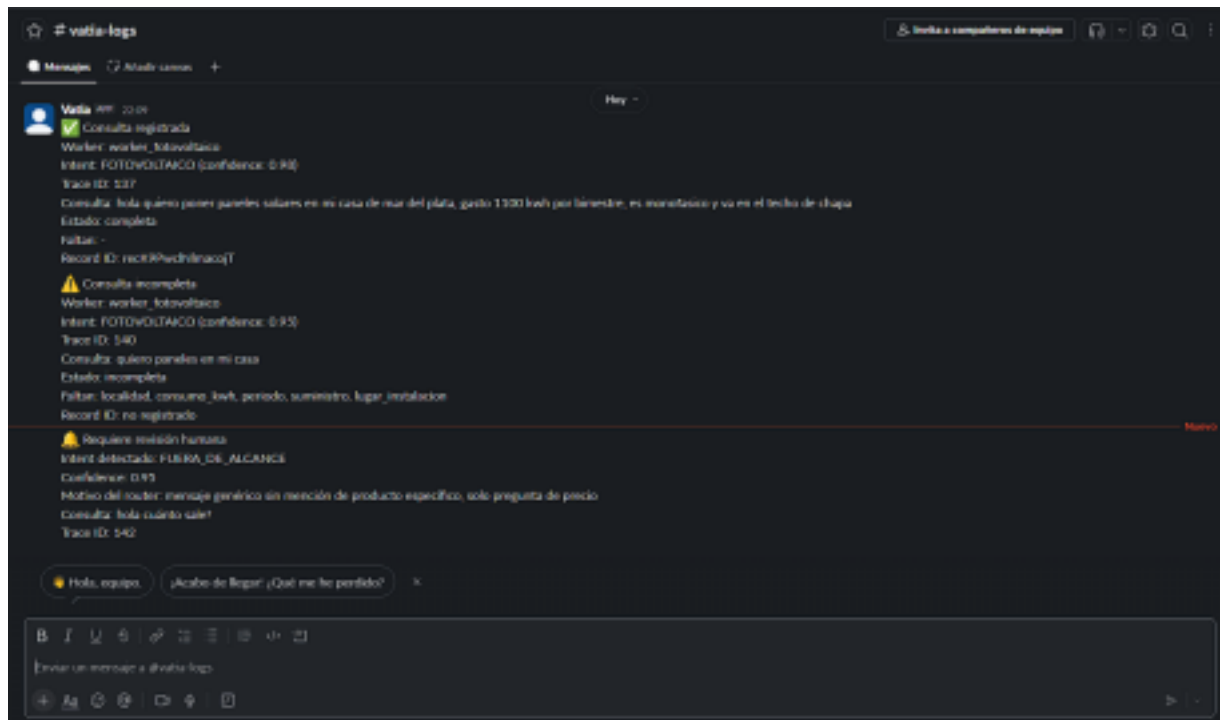
Figura 8 — Canal #vatia-logs. Los tres caminos posibles del sistema en una misma sesión de pruebas: consulta registrada con record_id (trace 137), consulta incompleta con el detalle de los campos faltantes (trace 140) y derivación a revisión humana con el motivo de la clasificación (trace 142).
