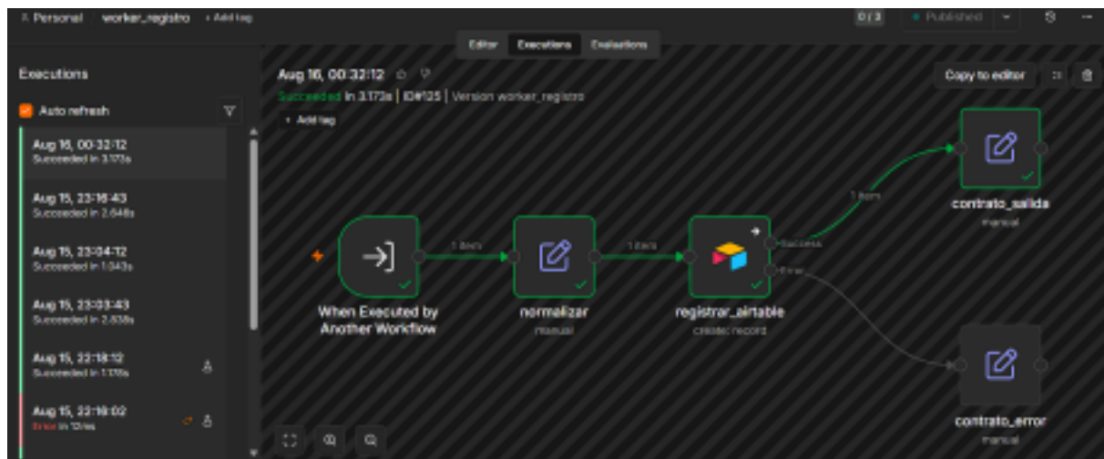
Figura 4 — worker_registro. Trigger → normalizar (Set) → registrar_airtable, con dos salidas: Success hacia contrato_salida y Error hacia contrato_error.
