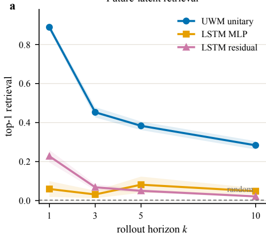
Future-latent retrieval
