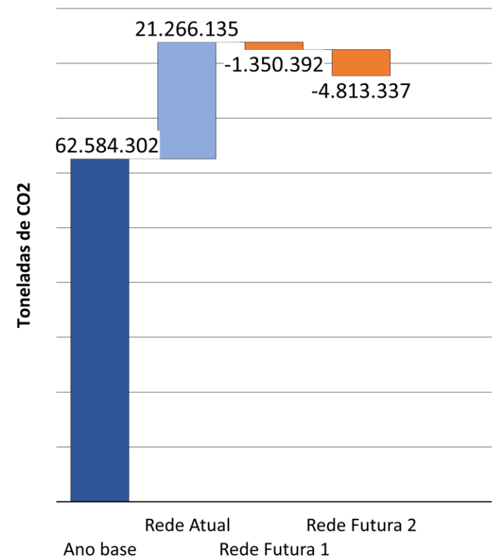
Evolução das emissões de CO 2 na sequência de cenários de rede
