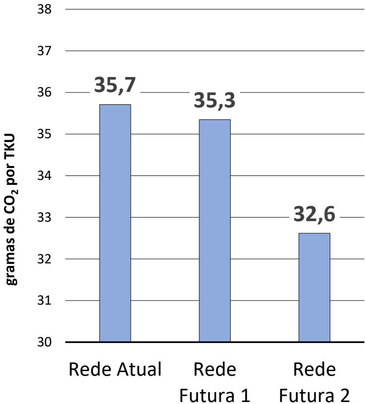
Emissões médias de CO 2 / TKU nos distintos cenários da rede em 2035
