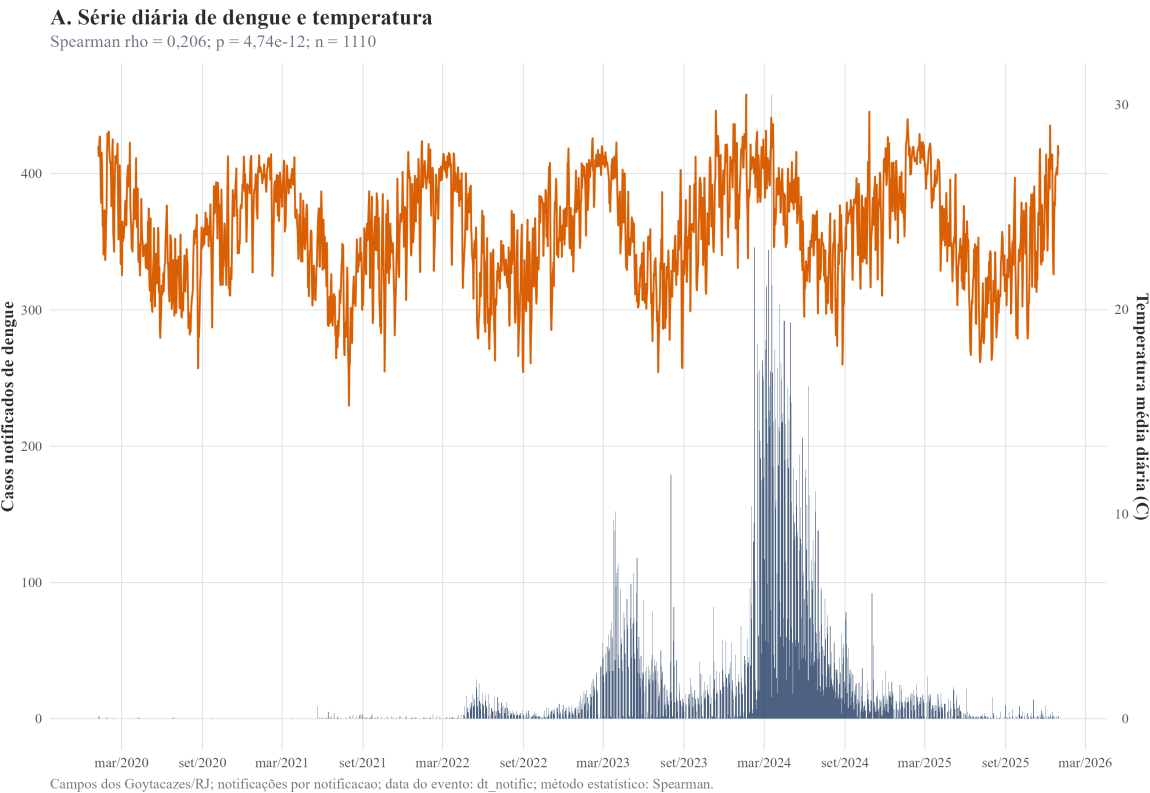
Figura 1 - Série diária de dengue e temperatura
