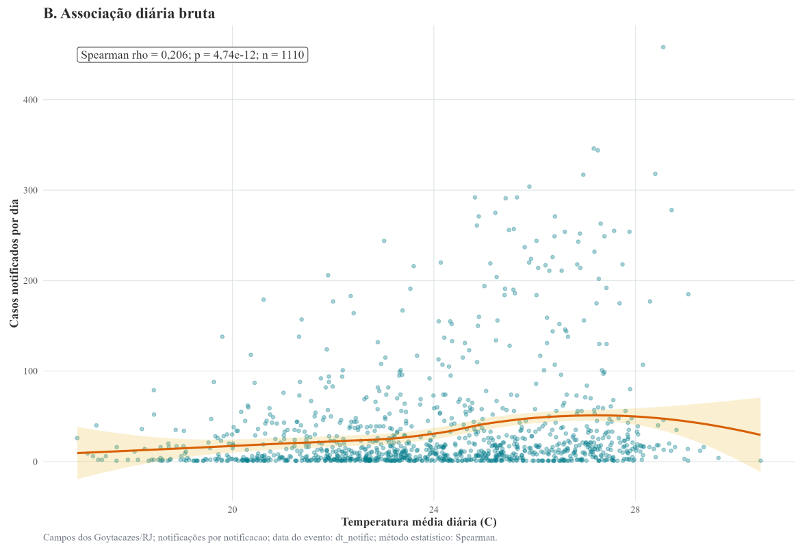
Figura 2 - Associação diária bruta
