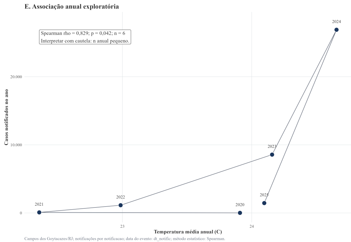
Figura 5 - Associação anual exploratória
