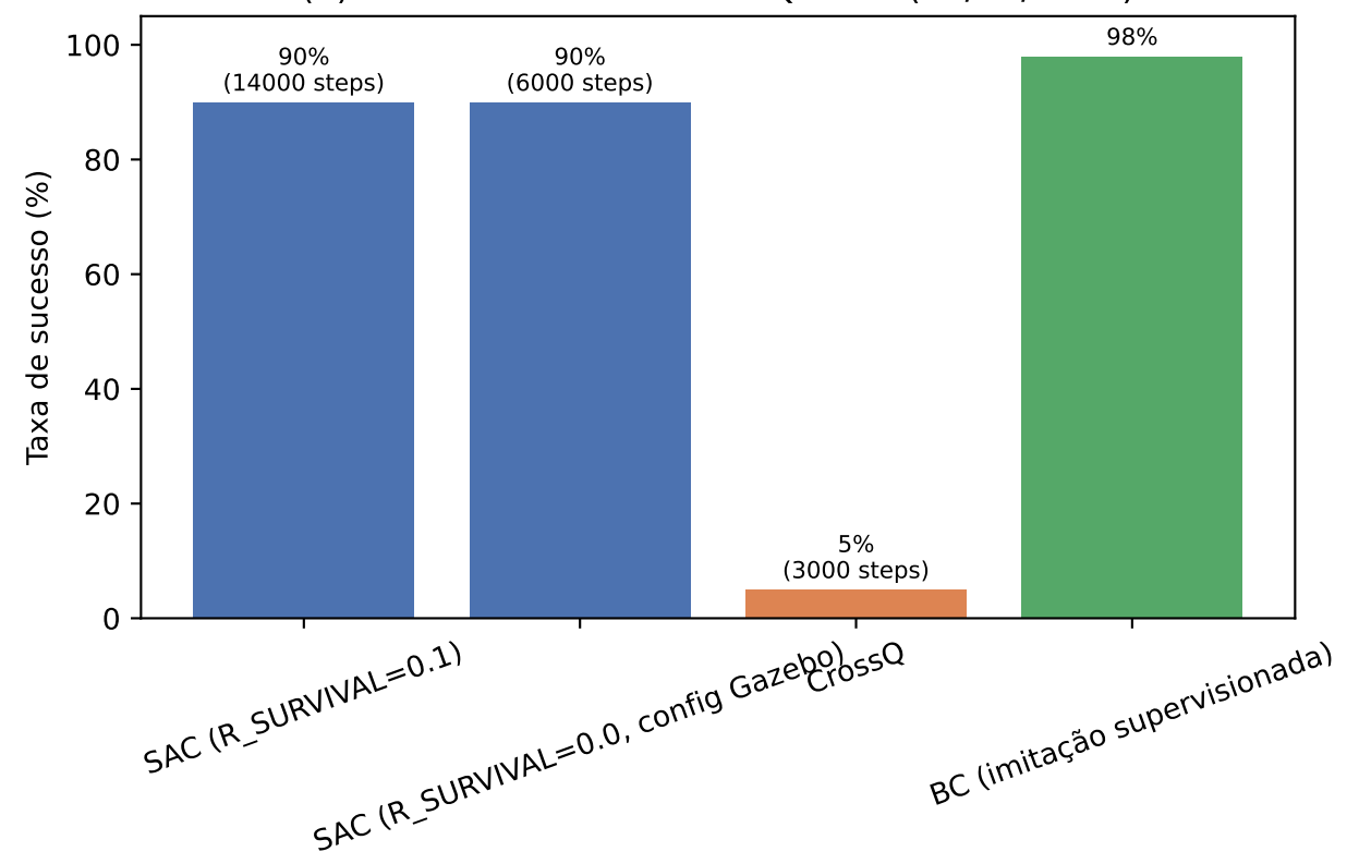
(d) 2D twin — SAC × CrossQ × BC (09/07/2026)
