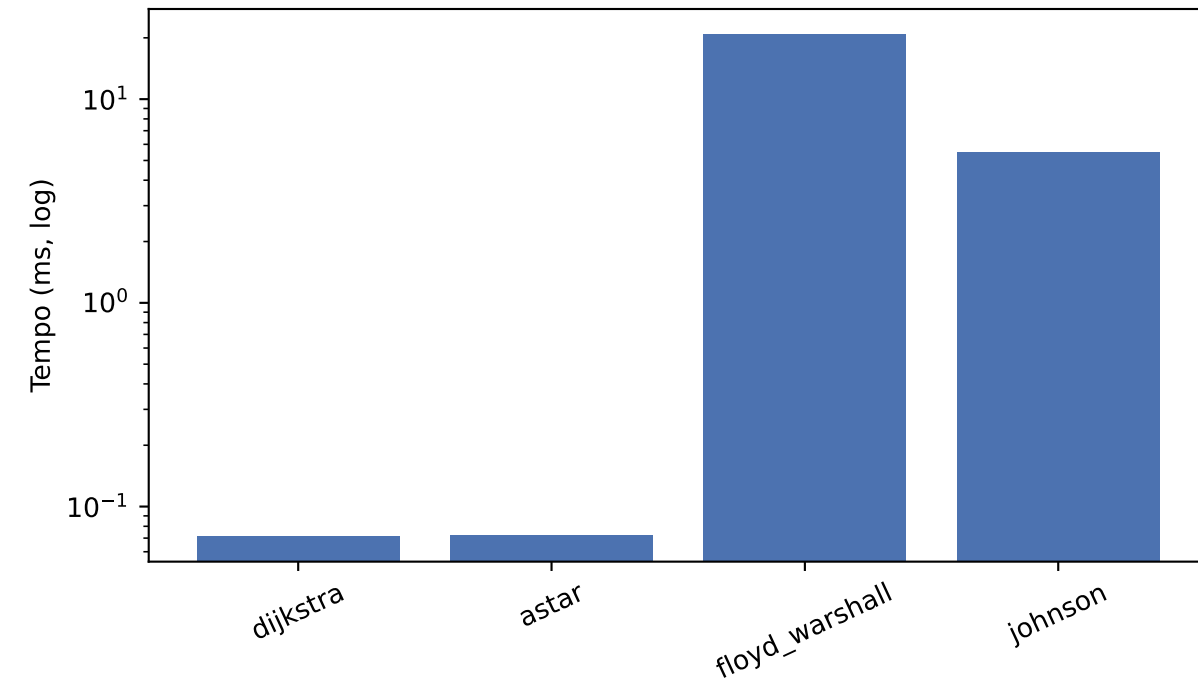
(a) Algoritmos clássicos — 100 nós (real)
