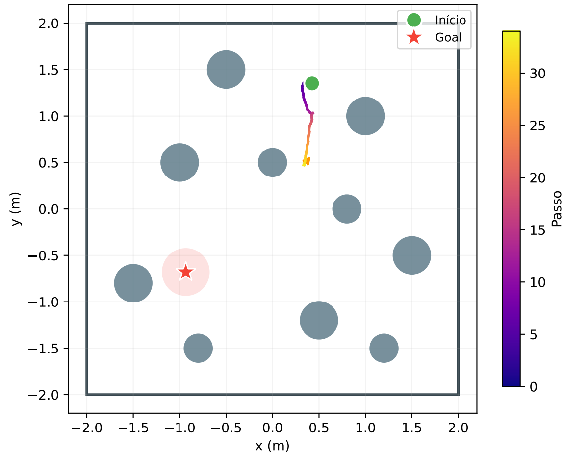
Trajetória SAC — env 2D (dense) 34 passos | reward=-89.3 | ✗ Colisão
