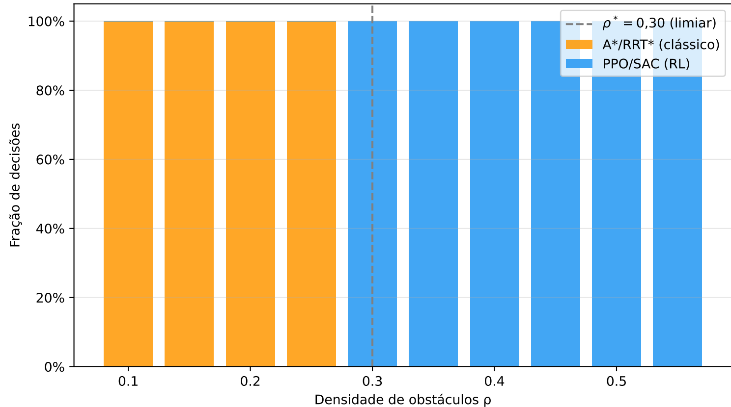
Distribuição de uso: clássico vs RL por densidade ( \tau=0,30 )
