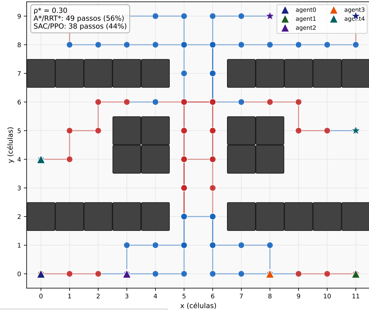
Decisão adaptativa por passo (azul = A*/RRT* | vermelho = SAC/PPO)
