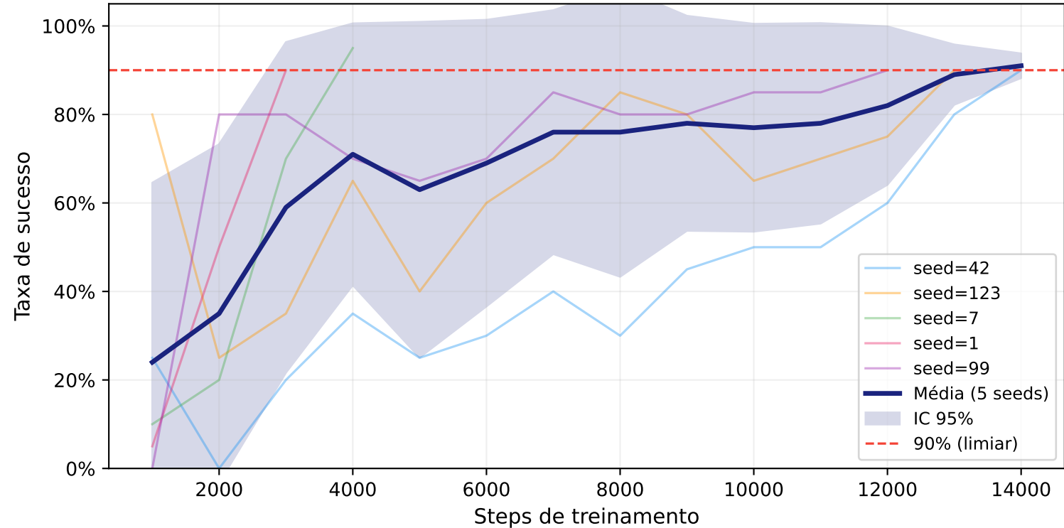
Curva de Aprendizagem SAC — Env 2D (5 seeds independentes) world=sparse, MAX_STEPS=200, R_APPROACH=10
