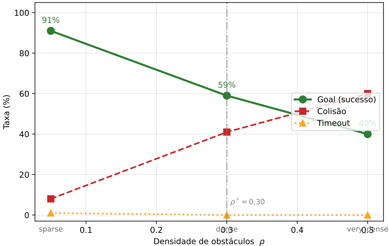
Degradação do SAC single-robot vs densidade (modelo treinado só no 'sparse', não generaliza)
