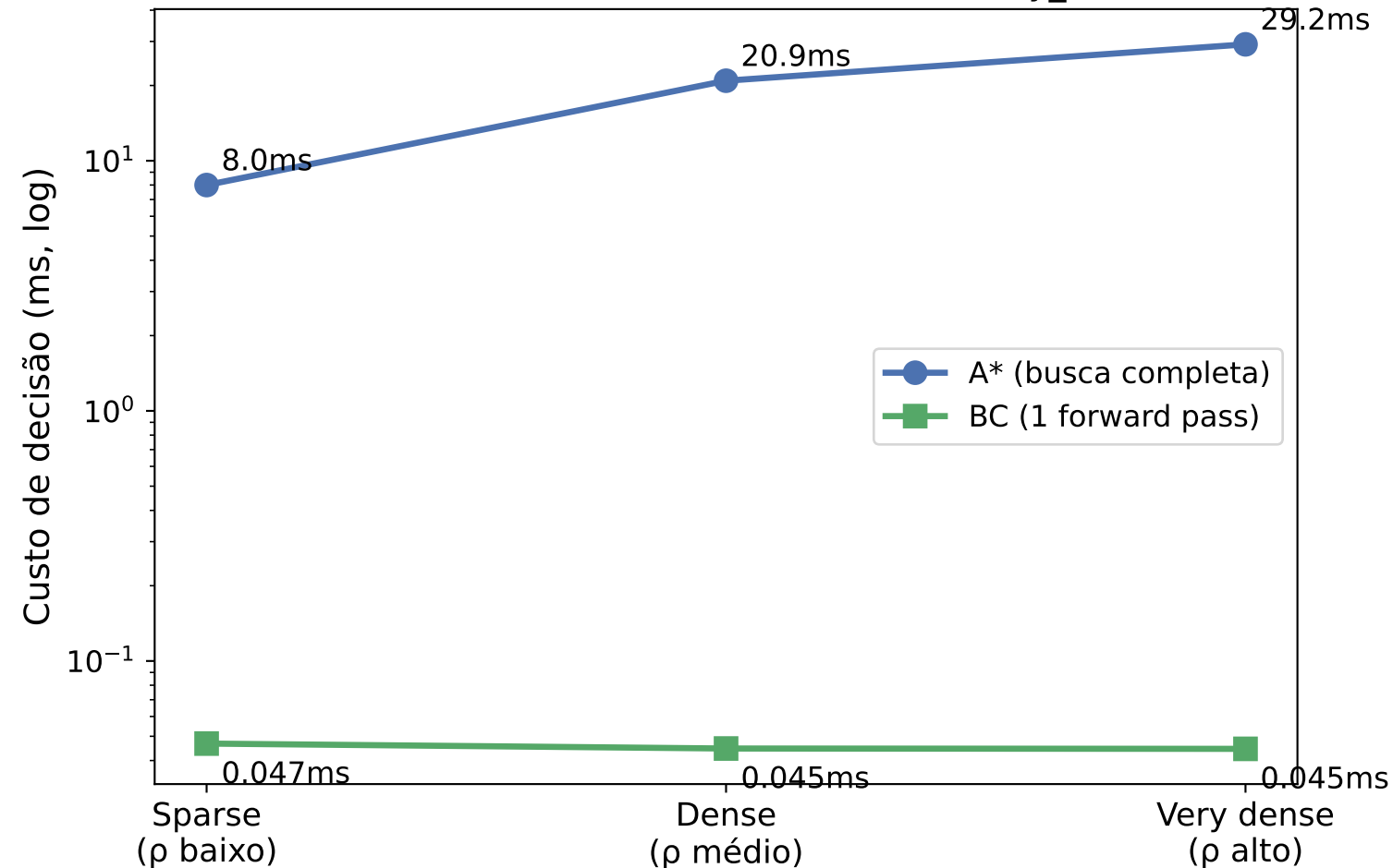
(b) Custo — BC ~656x mais barato em very_dense
