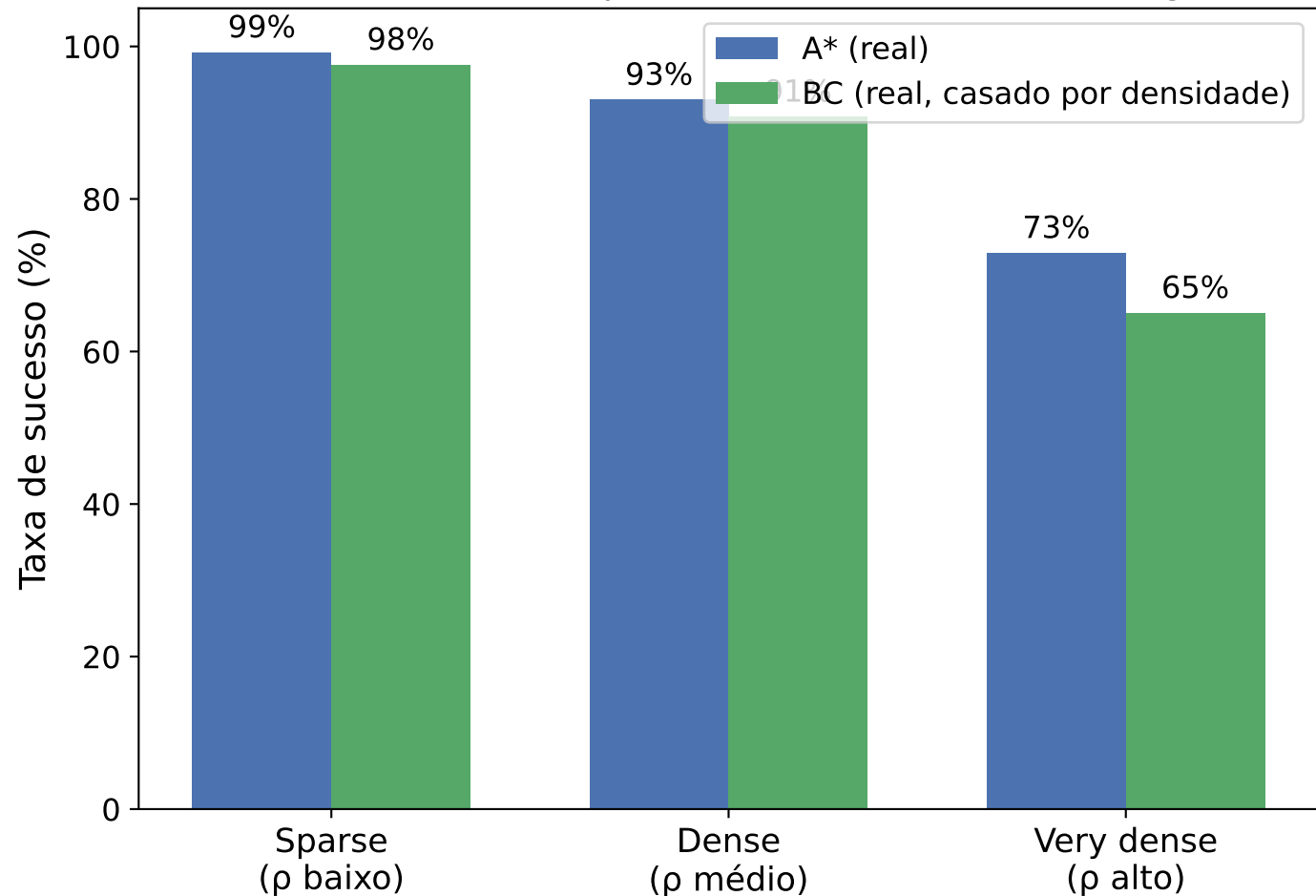
(a) Sucesso — A* real permanece à frente em todo regime
