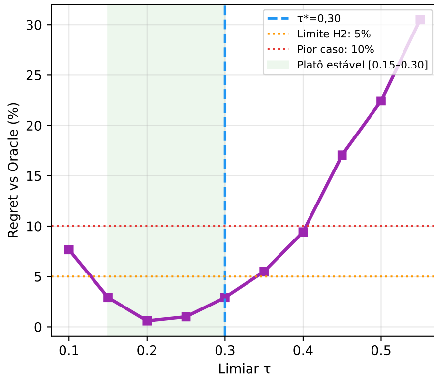
(b) Regret — \tau=0,30 na borda do platô
