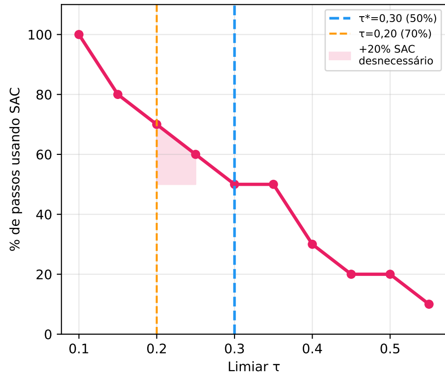
(a) Uso de SAC diminui com \tau maior
