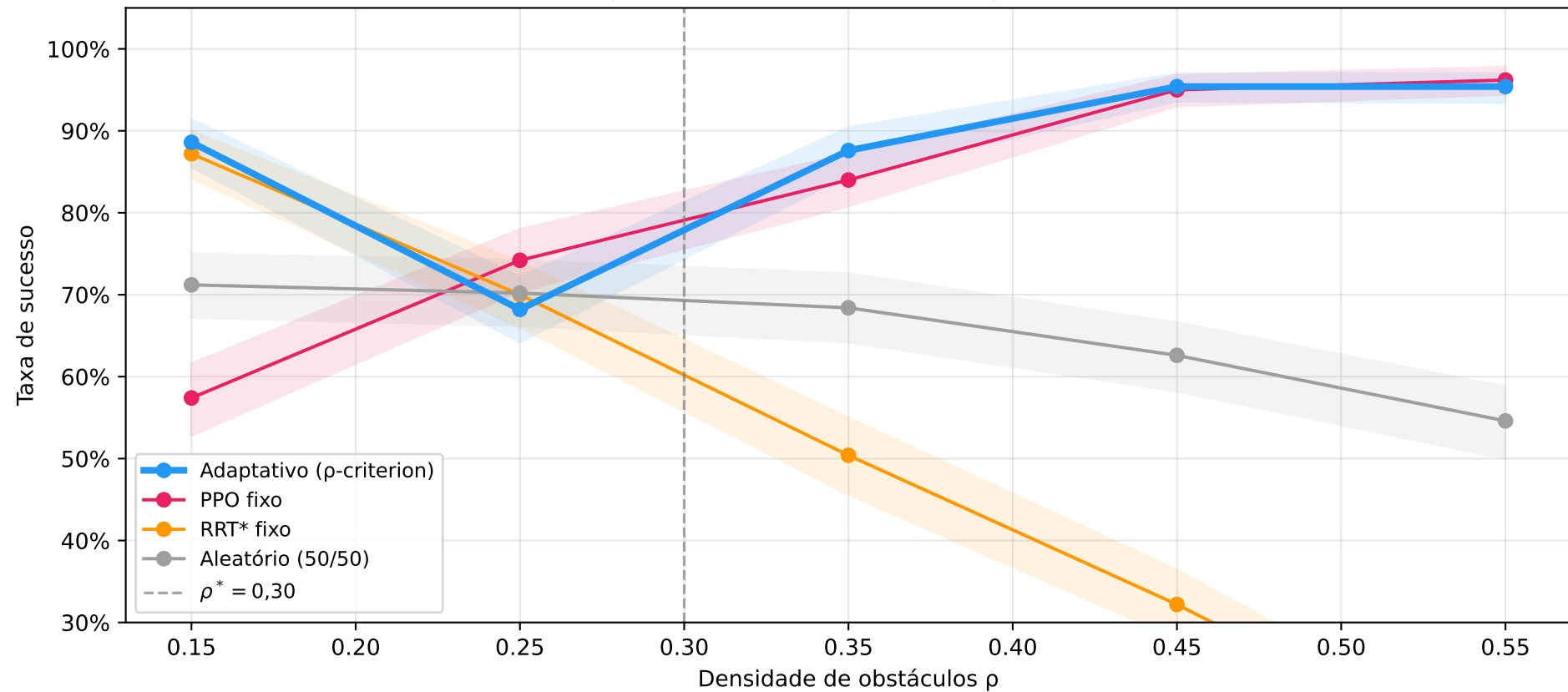
Taxa de sucesso — N=500 trials/densidade, IC 95% Adaptativo vs PPO fixo: z=5.51 , p=0.0000^*
