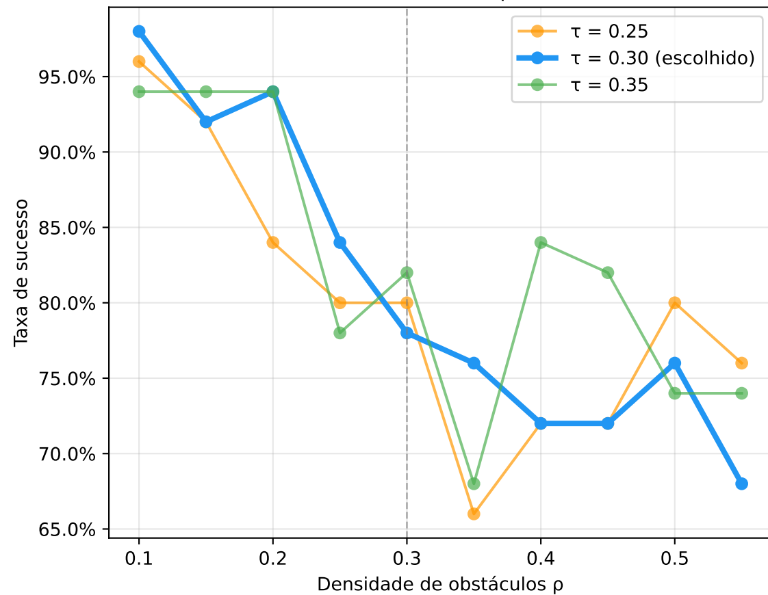
Sensibilidade ao limiar \tau por densidade
