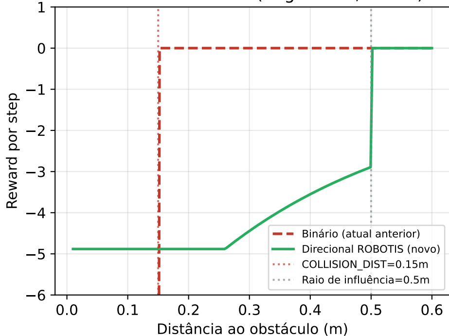
Obstacle Reward Direcional — padrão-ouro ROBOTIS (2021) direcional \cos(\theta)^6 Reward vs distância (ângulo=0°, frente) antes da colisão vs penalidade (frente=1, lateral=mín)
