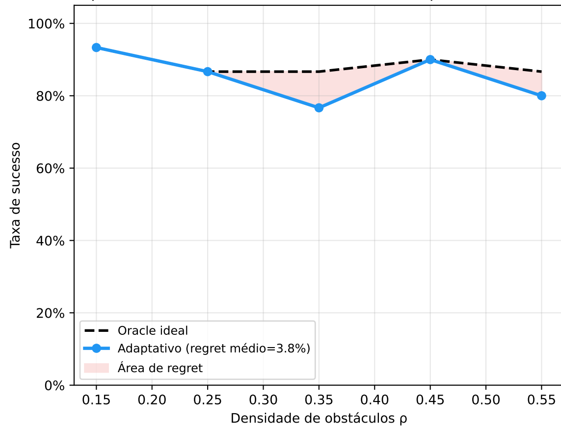
\rho -criterion vs Oracle — distância ao desempenho máximo
