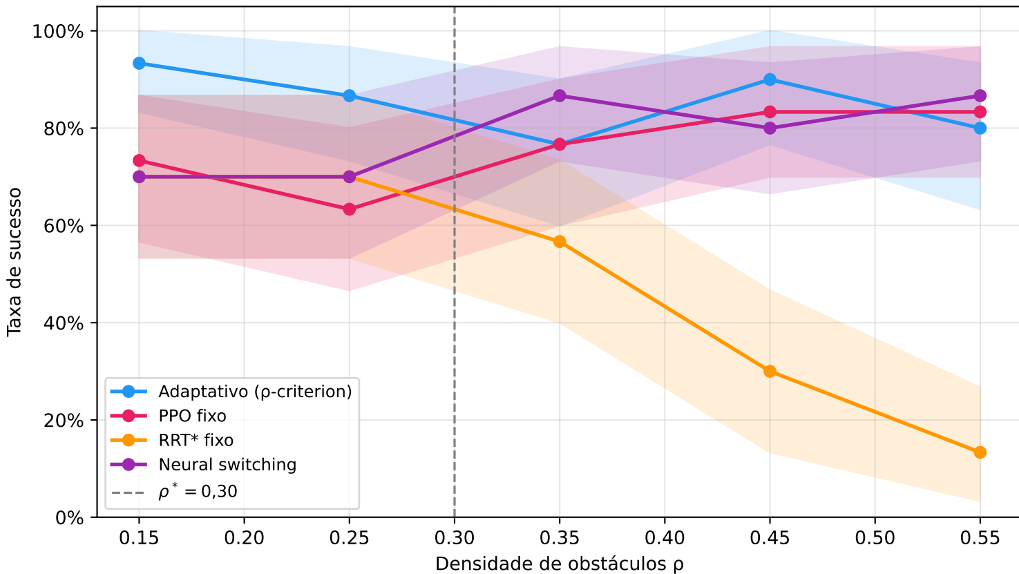
Taxa de sucesso por densidade — IC 95% (bootstrap binomial) z = 2.05 , p = 0.020^* vs PPO fixo
