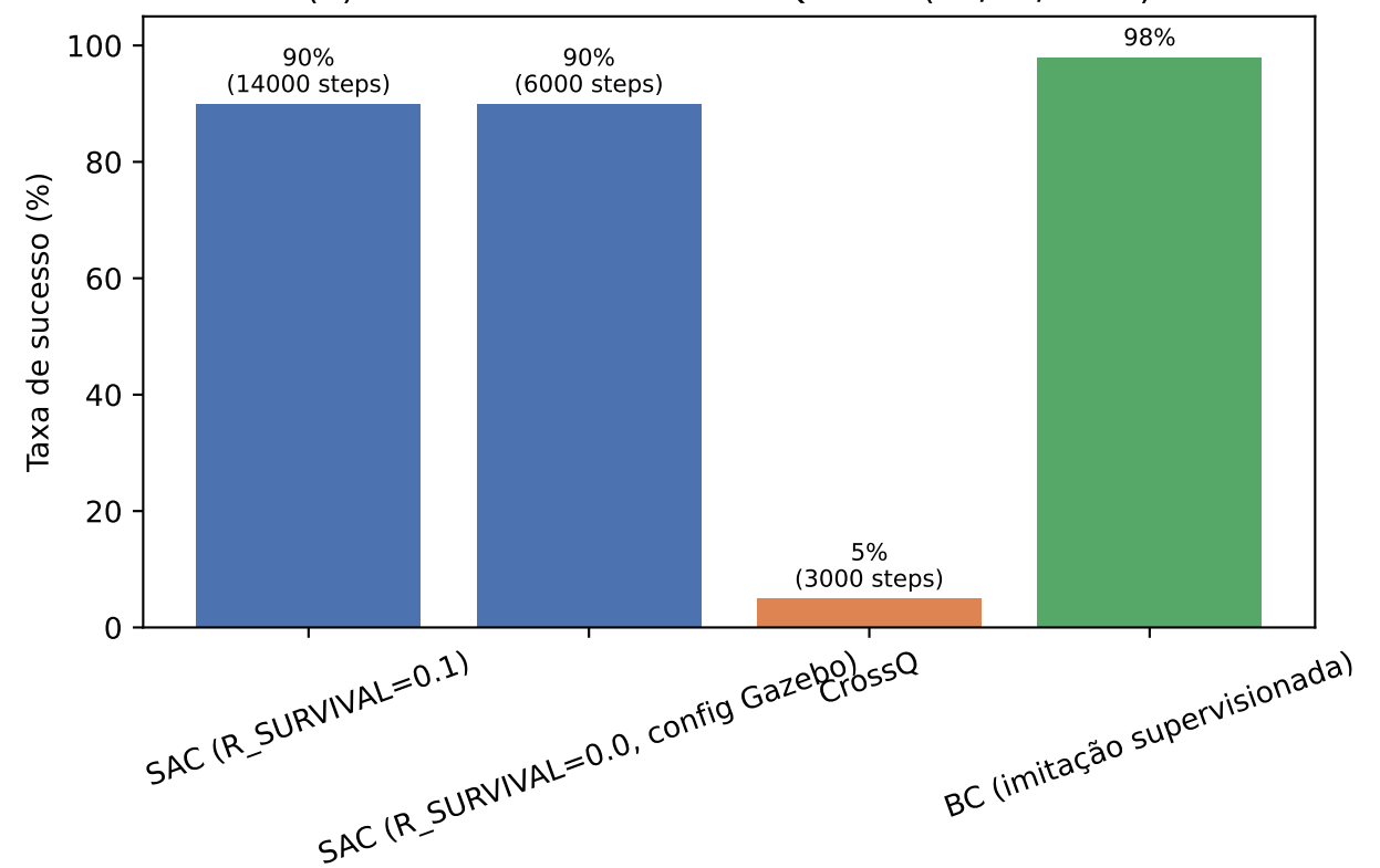
(d) 2D twin — SAC × CrossQ × BC (09/07/2026)
