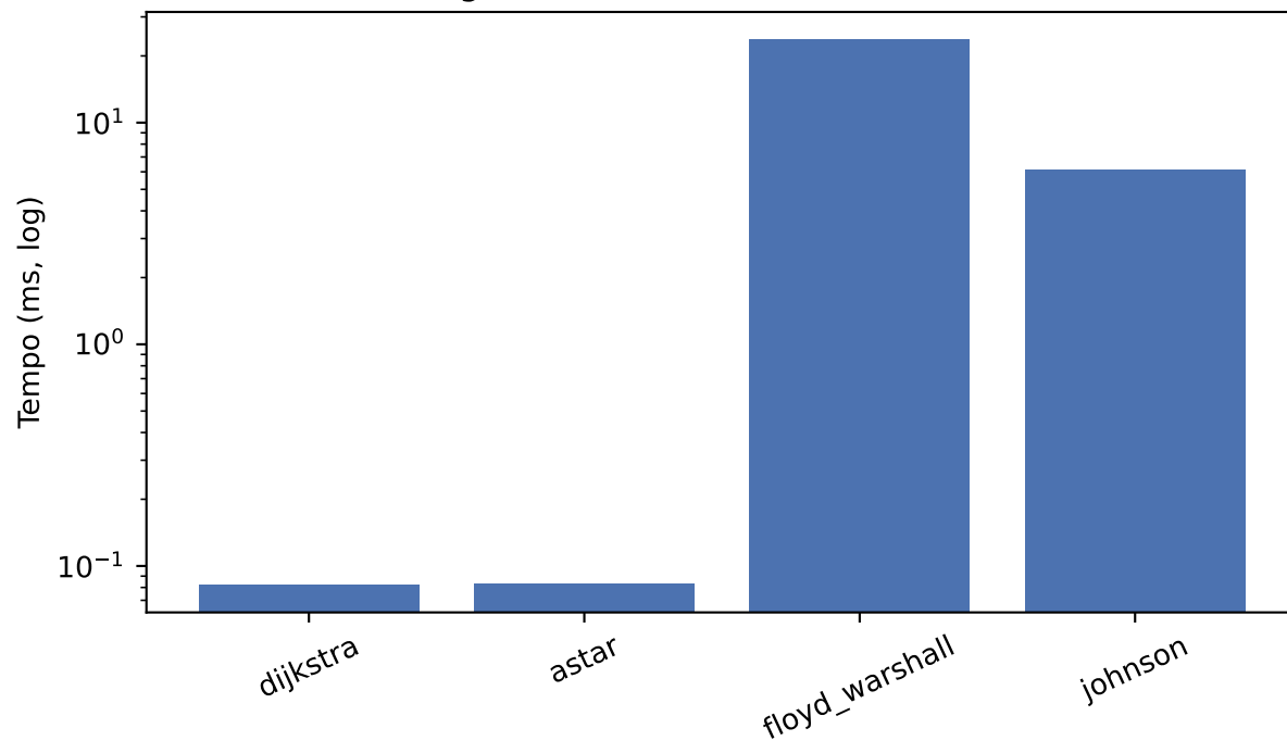
(a) Algoritmos clássicos — 100 nós (real)
